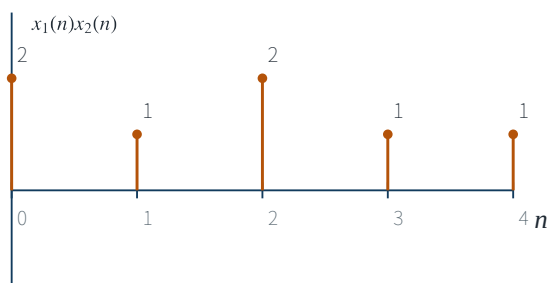
逐项相乘的结果
