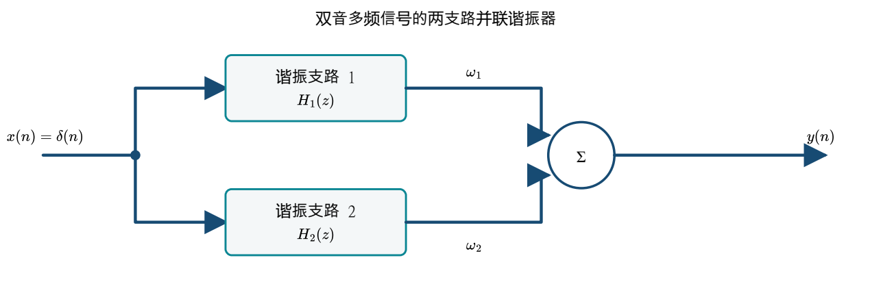
图 5-5 并联型结构示例：双音多频信号
