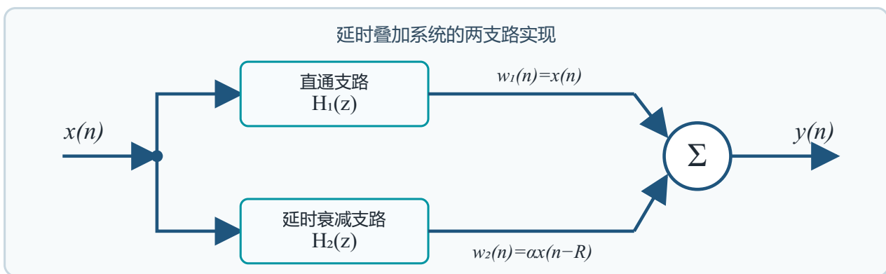
图 1-11 延时叠加系统的标准结构图：两条支路在求和器处汇合。
