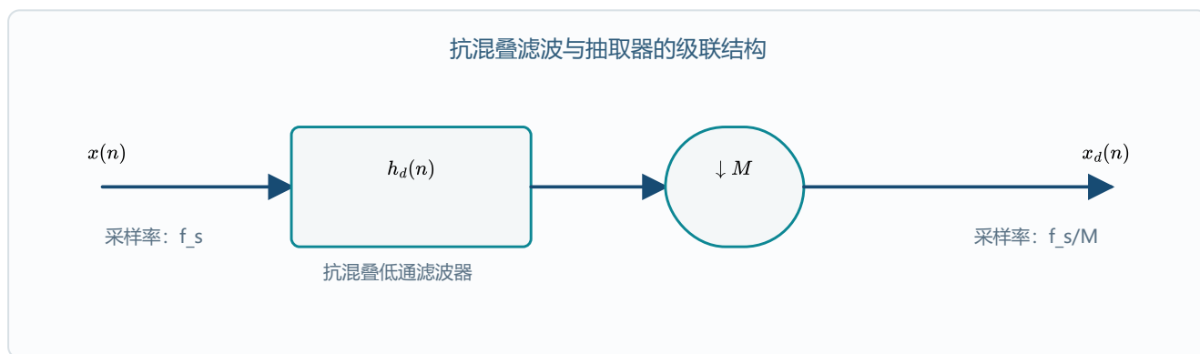
图 8-2 抗混叠滤波与抽取器的级联结构
