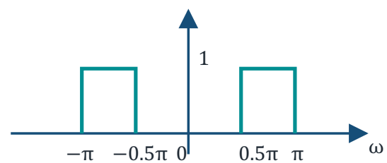
H(e^{j\omega}) 数字滤波器频率响应
