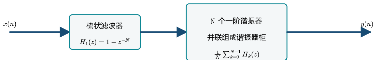
频率采样型 FIR 的梳状滤波器与谐振器柜
