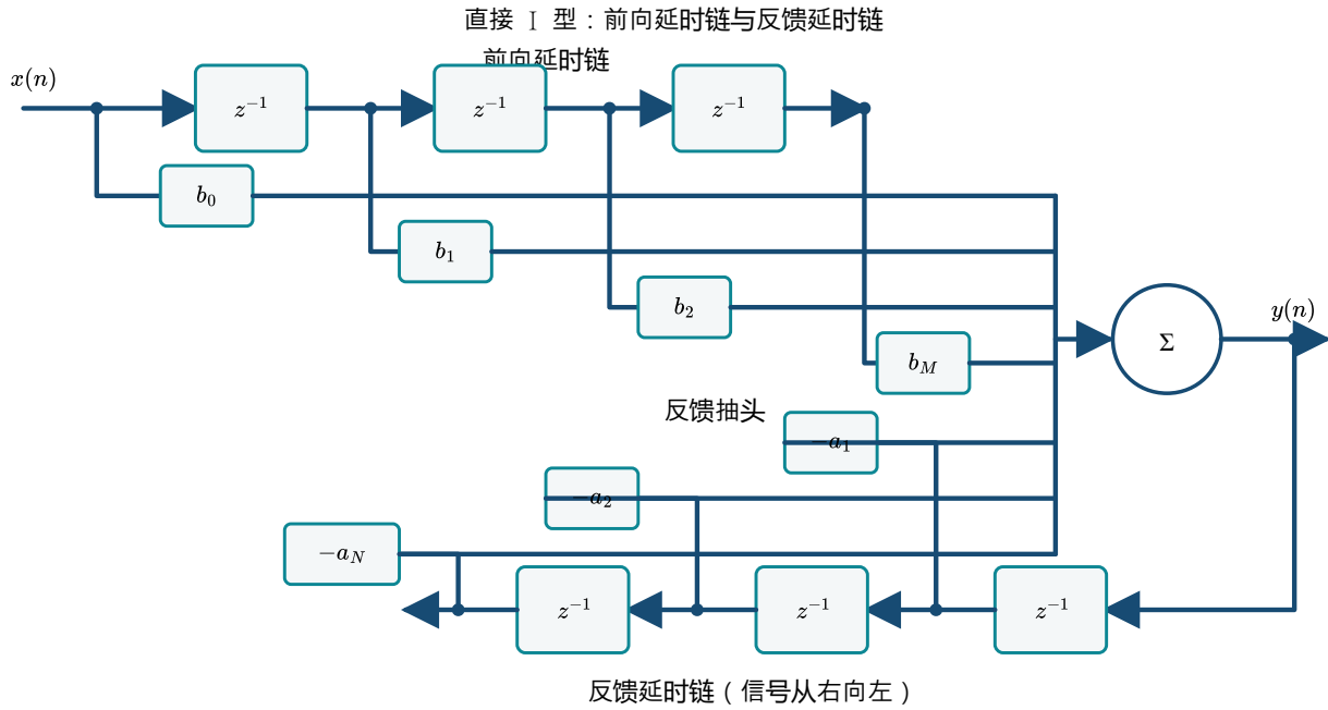
图 5-1 IIR 直接 I 型结构
