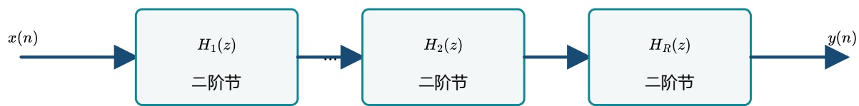
IIR 二阶节级联结构
