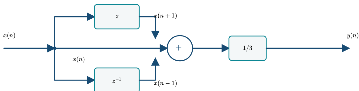
原三抽头平均器：含超前项，故非因果
