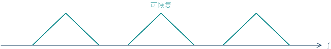
先限制输入带宽：频谱副本分离
