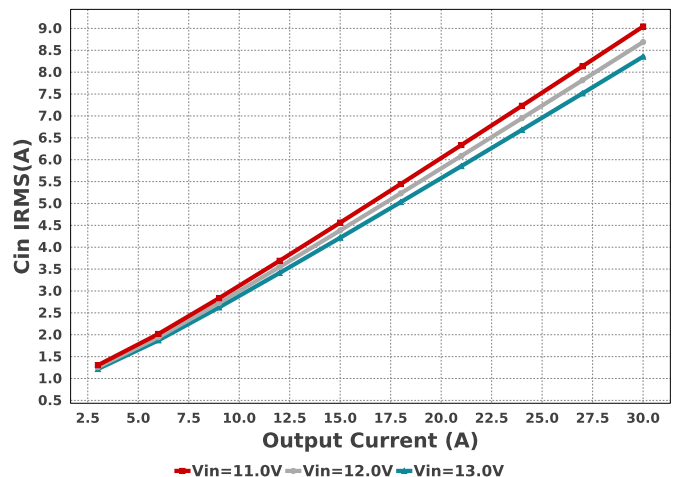
Cin IRMS
