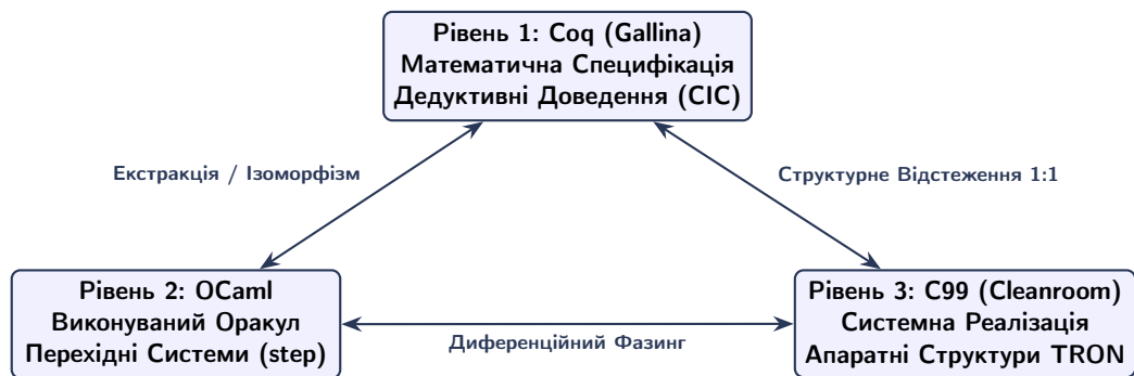
Рис. 2: Трикутник відстежуваності: математична специфікація, виконуваний оракул та код C99.
