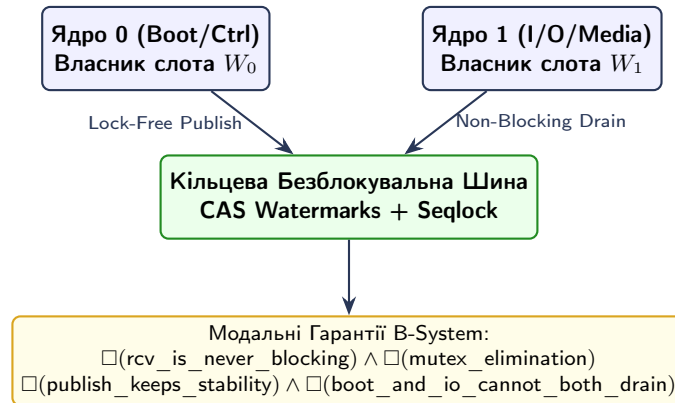
Рис. 1: Модальна багатоядерна модель B-System: ізоляція слотів та доведена ліквідація блокувань.
