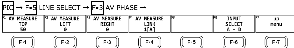
Figure 13-37 AV PHASE menu
