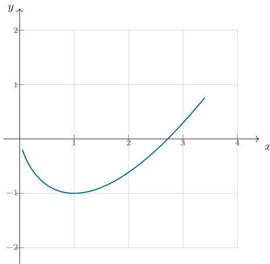
C_f : y = x \ln x - x — minimum -1 en x = 1 , zéro en x = e .
