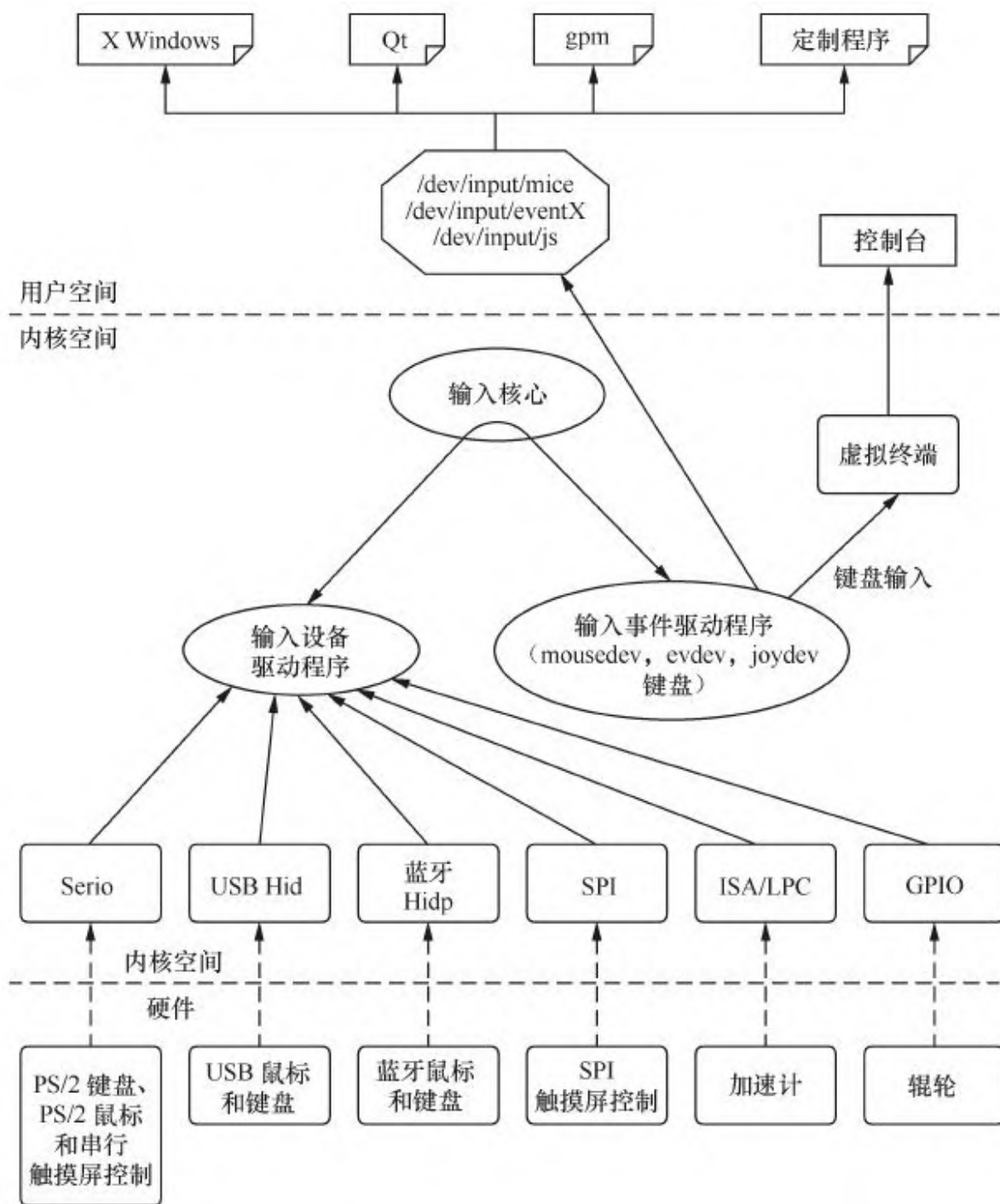
图12.6 Linux内核输入子系统的框架
