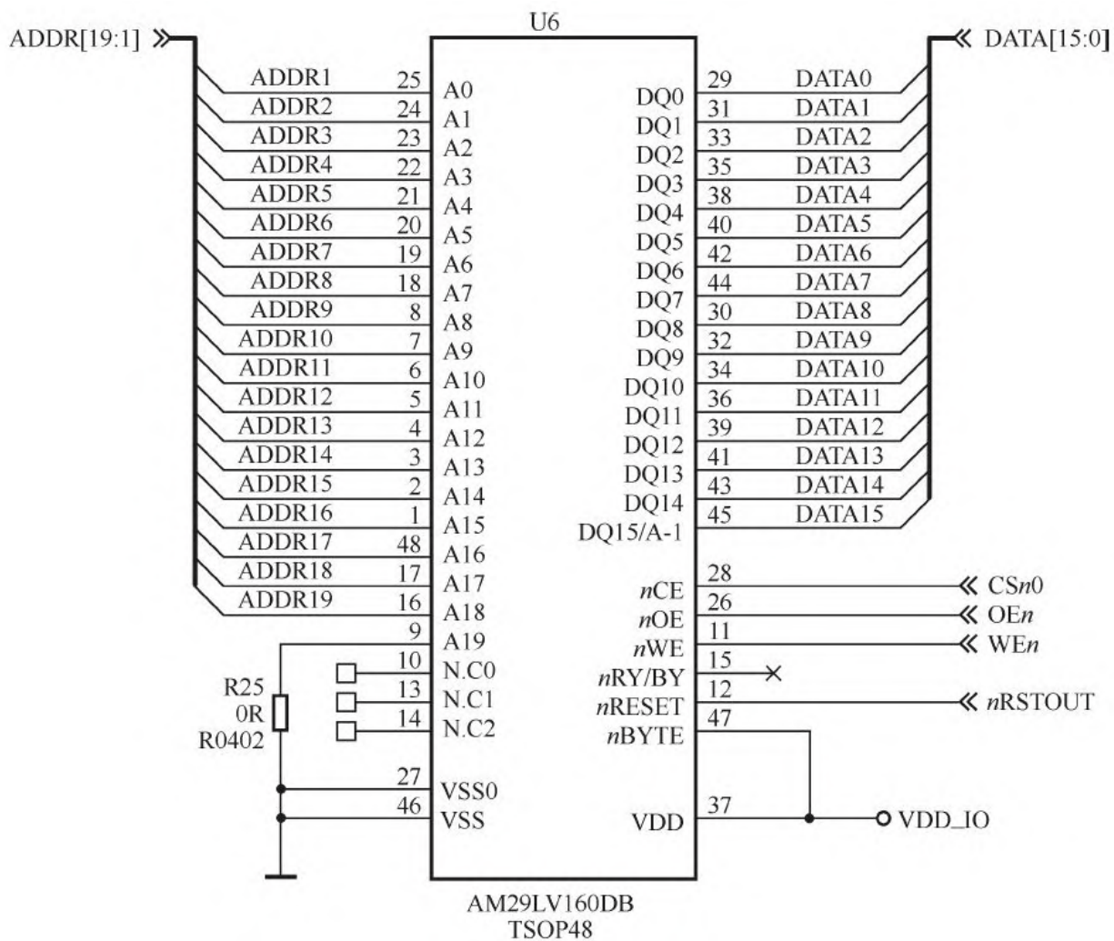
图2.23 原理图中的网络
