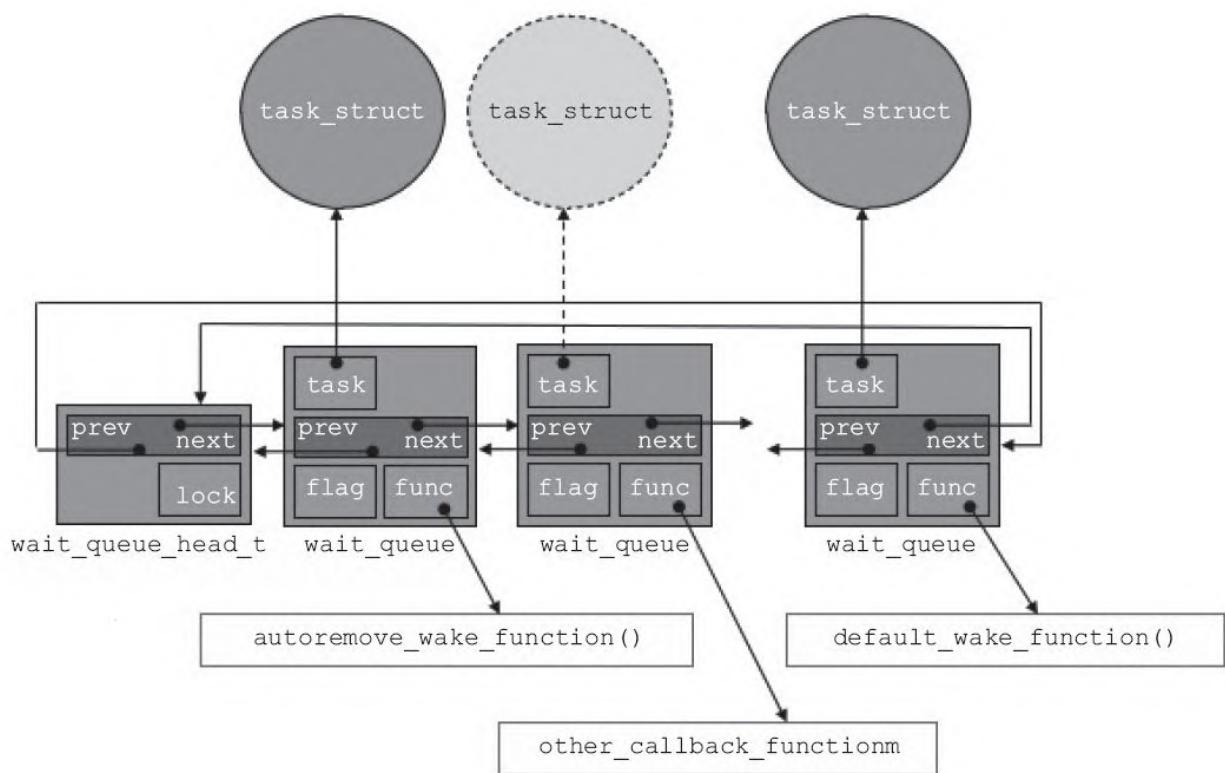
图8.2 wait_queue_head_t 、 wait_queue 和 task_struct 之间的关系
