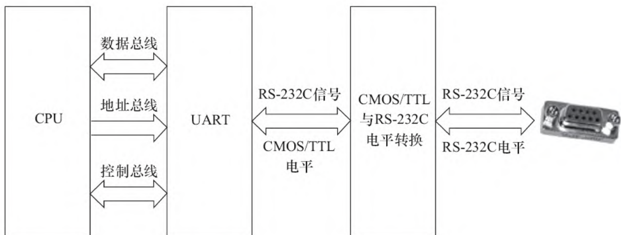
图2.9 RS-232C串口电路原理
