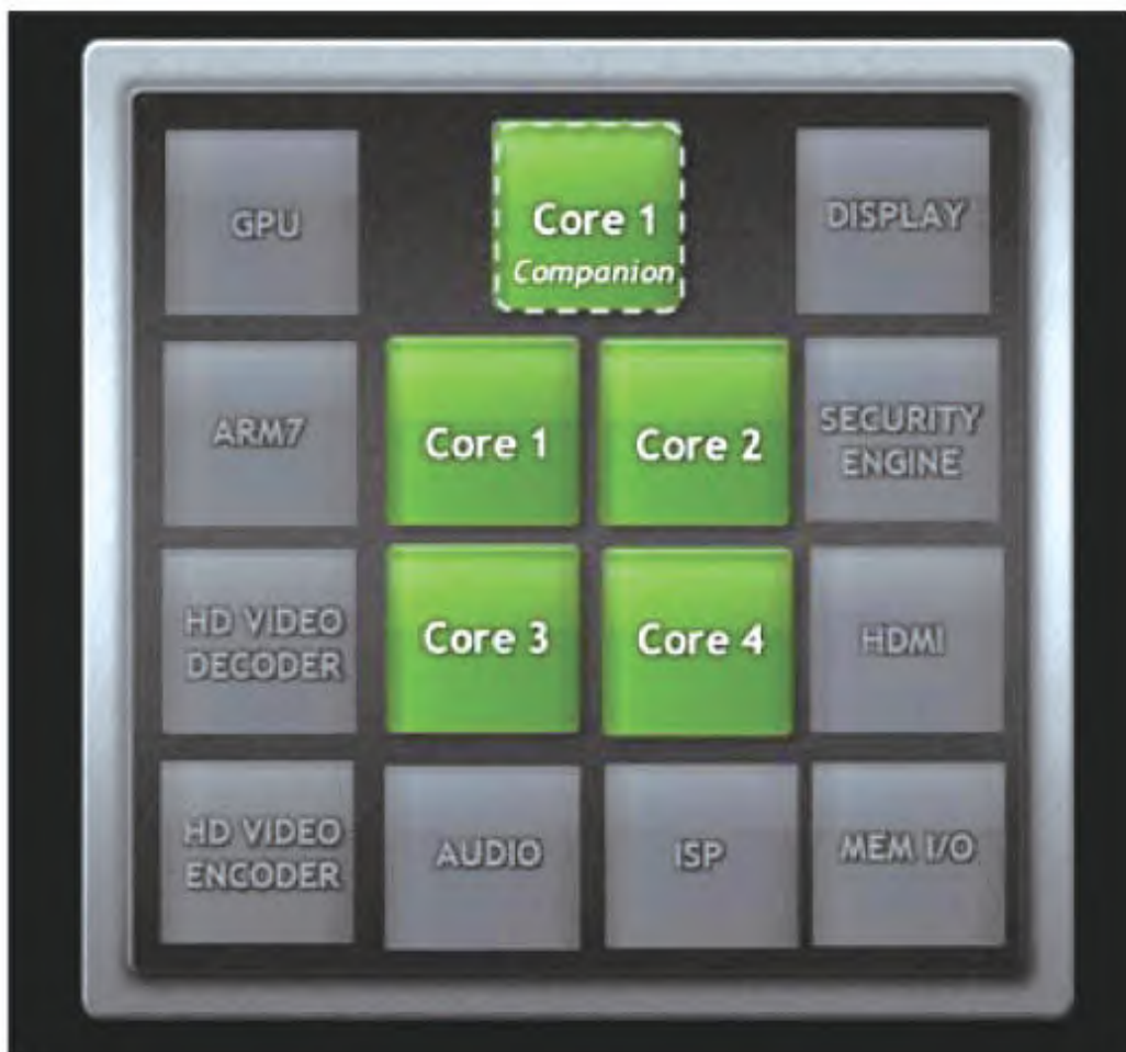
图19.7 Tegra3的架构
