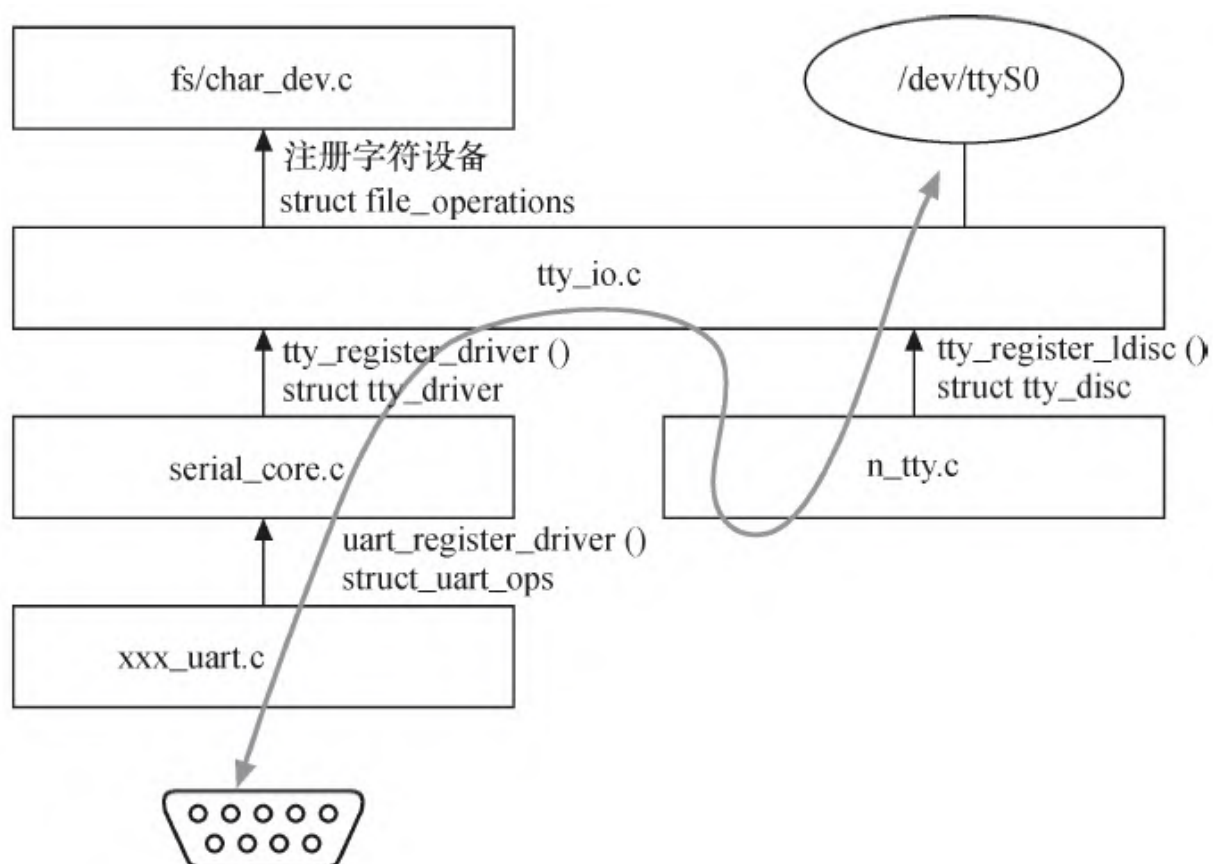
图12.11 串口核心层
