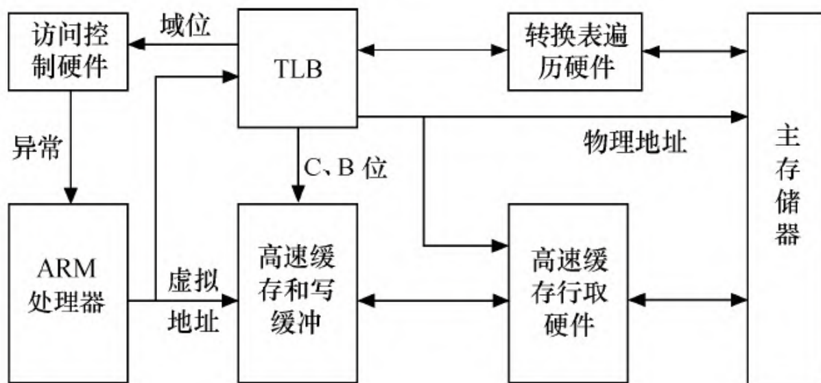
图11.3 ARM处理器的MMU
