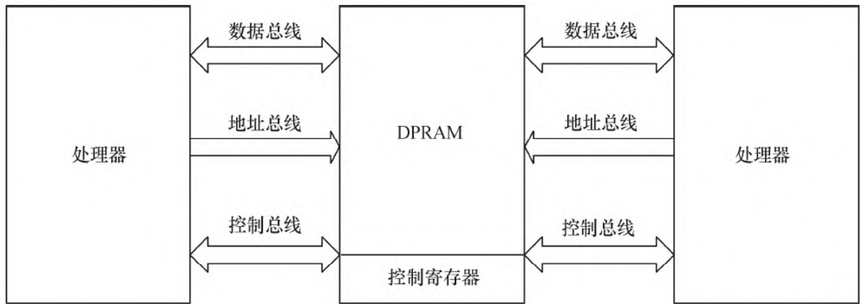
图2.6 双端口RAM
