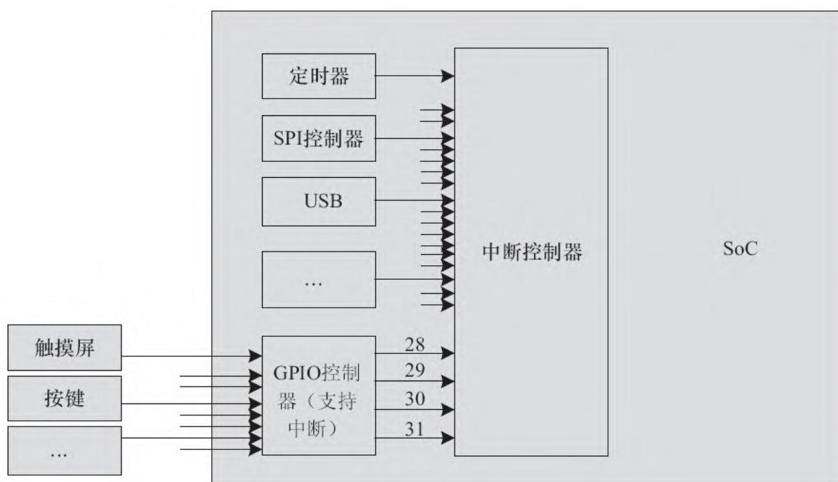
图20.4 SoC中断控制器的典型分布
