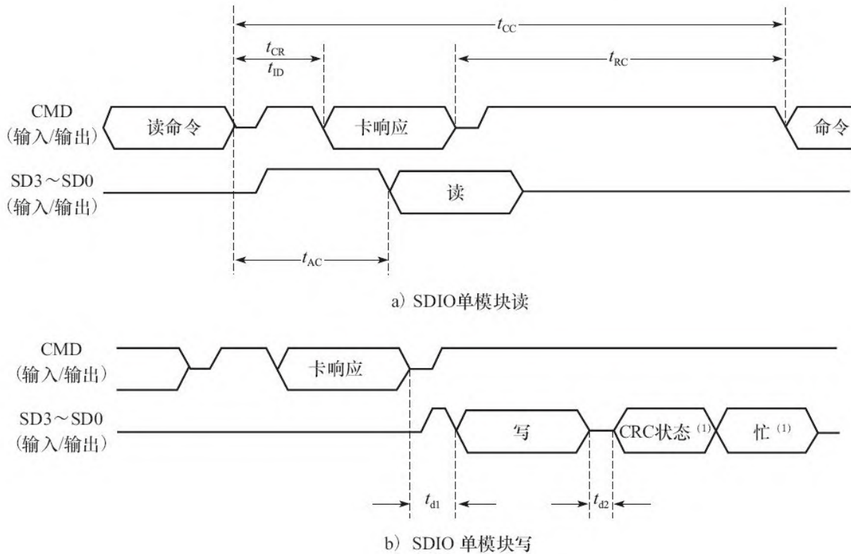
图2.18 SDIO单模块读、写的典型时序
