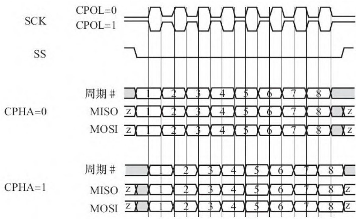
图2.13 SPI总线的时序
