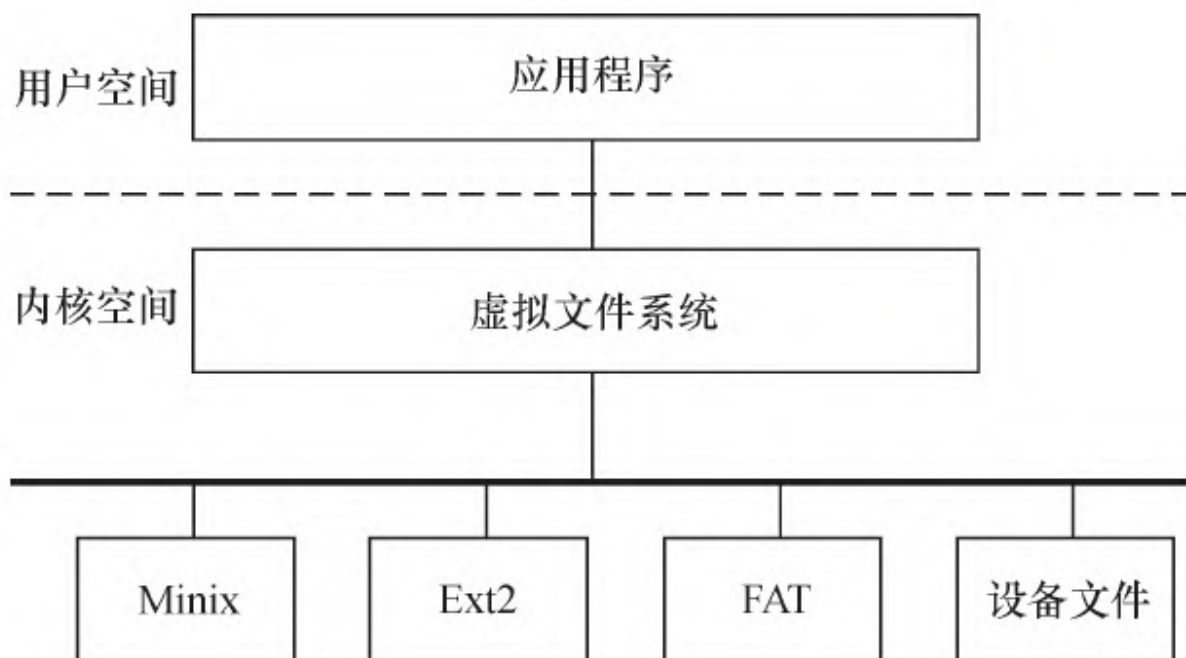
图3.7 Linux虚拟文件系统
