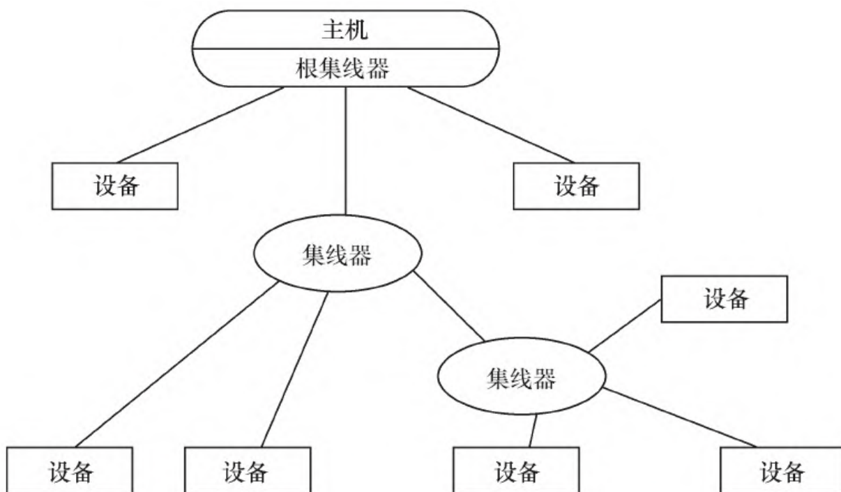
图2.14 USB的物理拓扑结构
