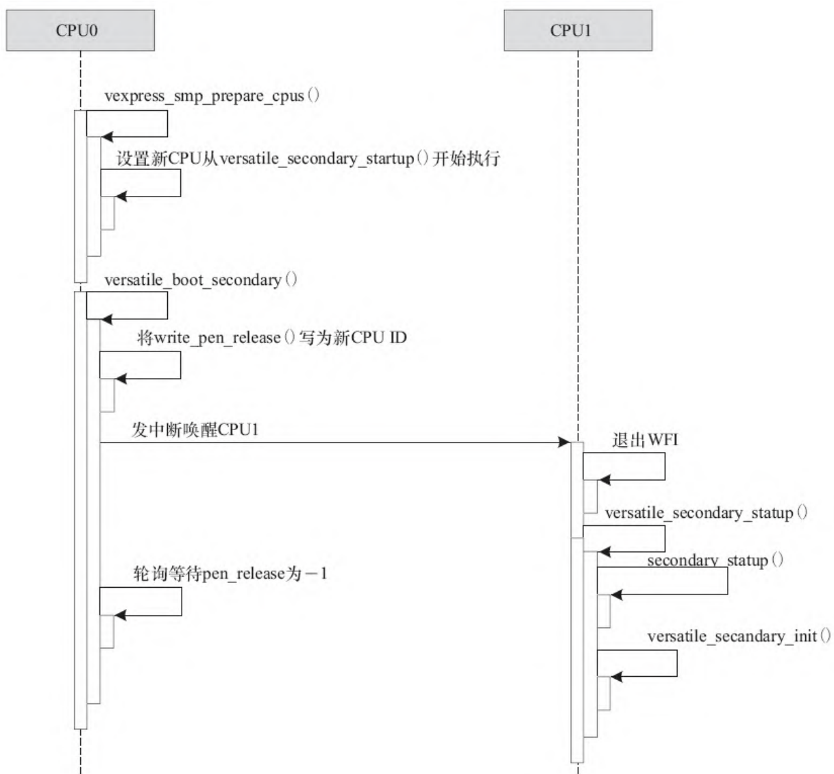
图20.7 CPU0唤醒其他CPU过程
