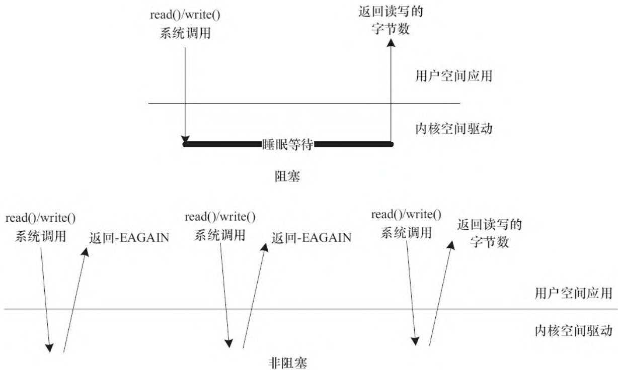
图8.1 阻塞与非阻塞I/O
