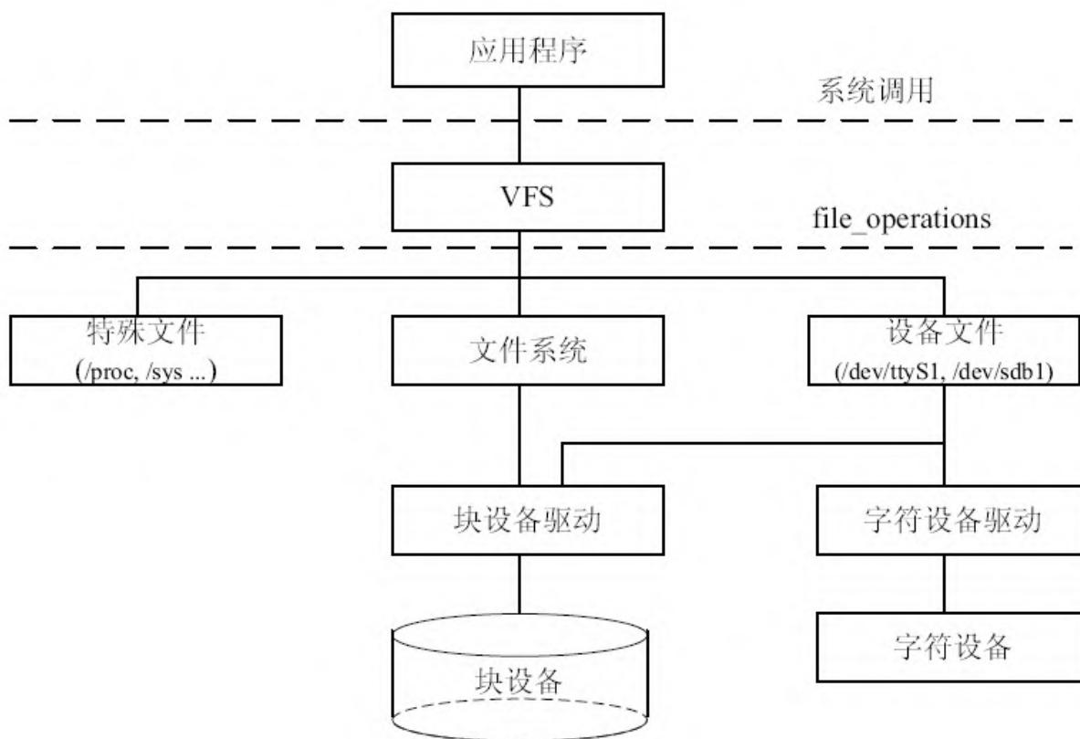
图5.1 文件系统与设备驱动之间的关系
