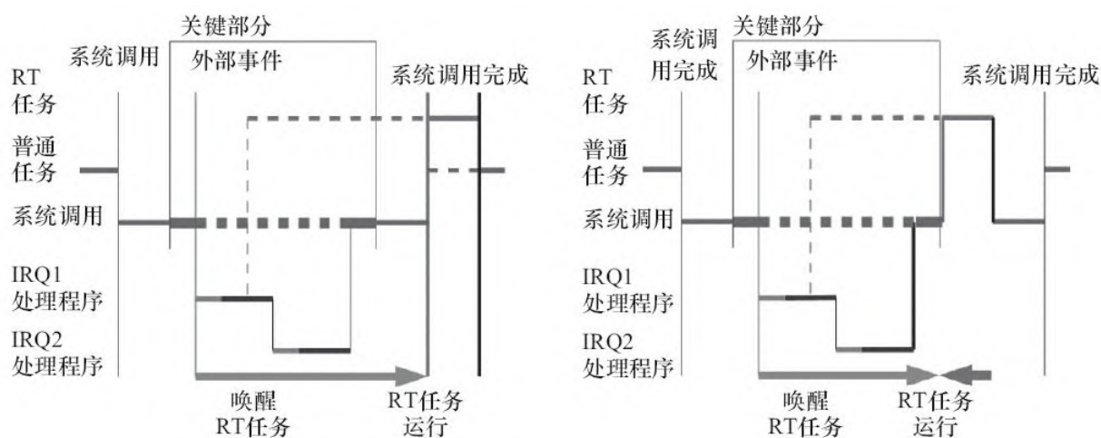
图3.2 Linux 2.4和2.6以后的内核在抢占上的区别
