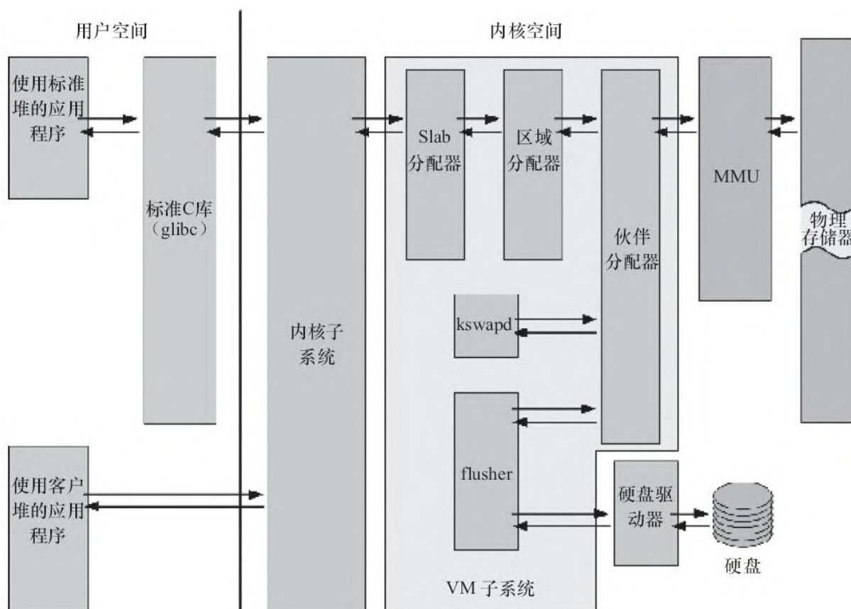
图3.6 Linux内存管理
