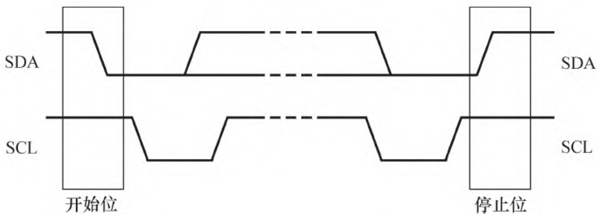
图2.10 I 2 C总线的开始位和停止位
