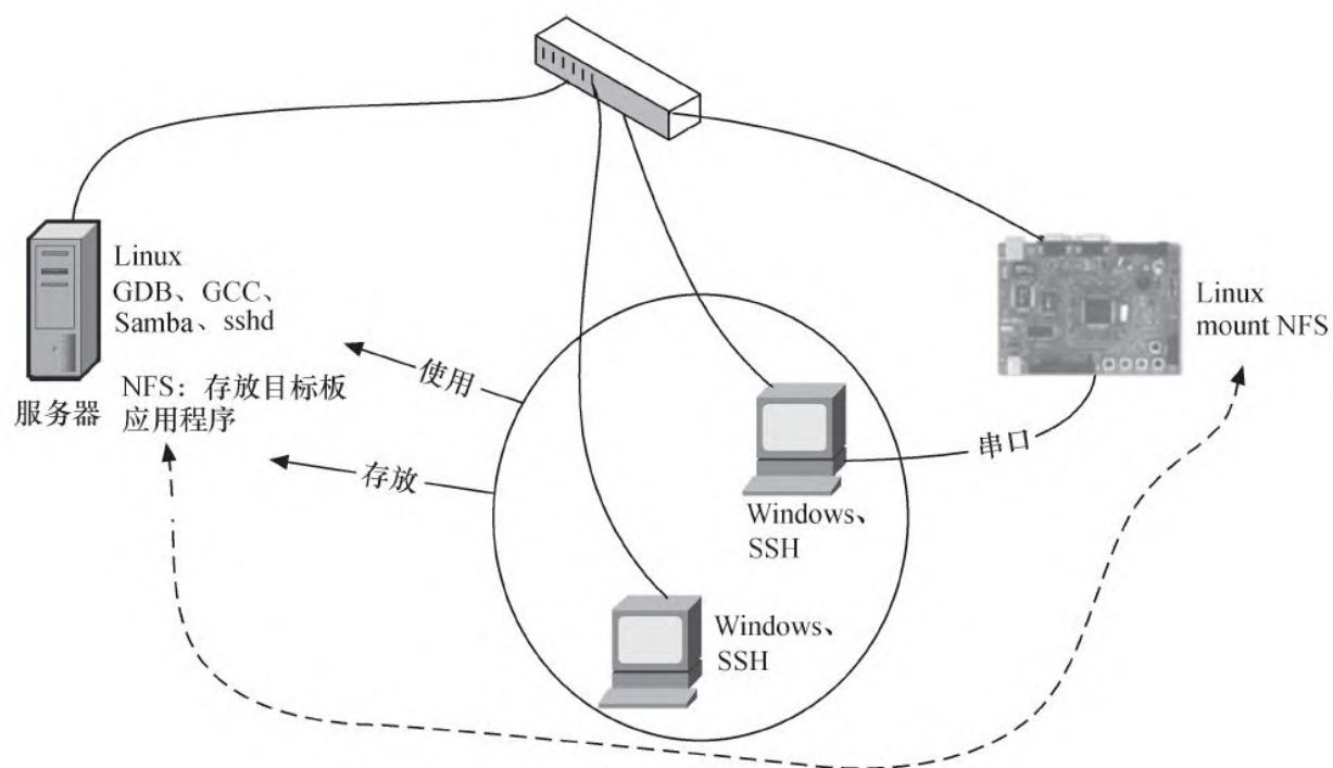
图3.13 小型Linux实验室环境
