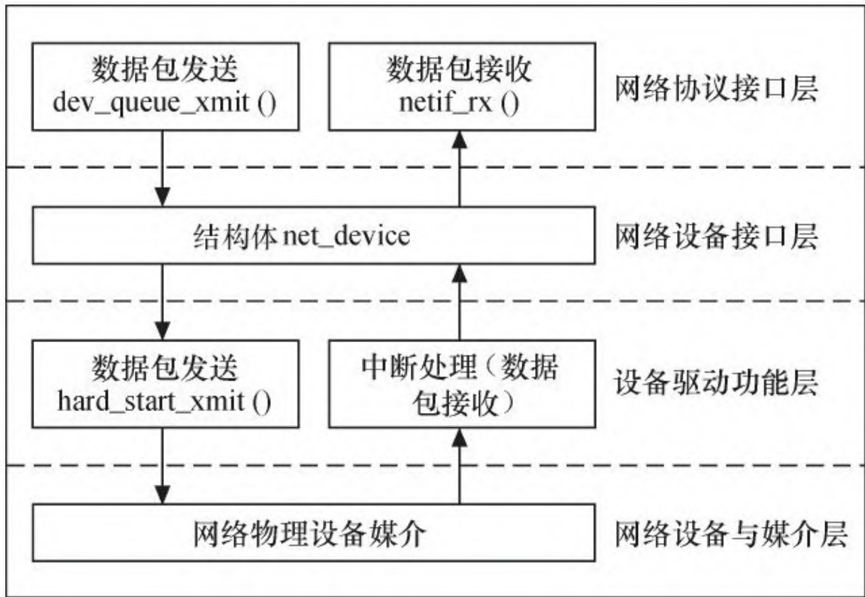
图14.1 Linux网络设备驱动程序的体系结构
