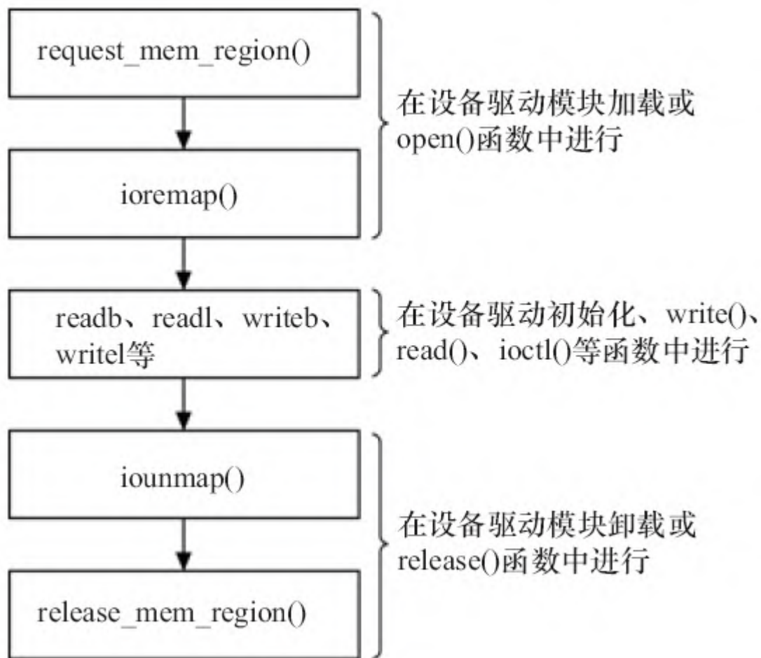
图11.11 I/O内存访问流程
