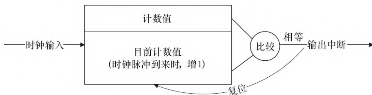
图10.1 PIT定时器的工作原理
