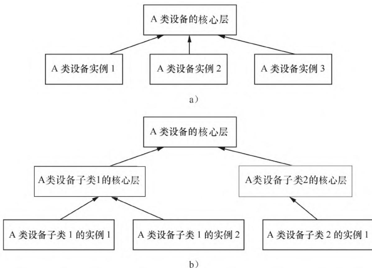
图12.5 Linux设备驱动的分层
