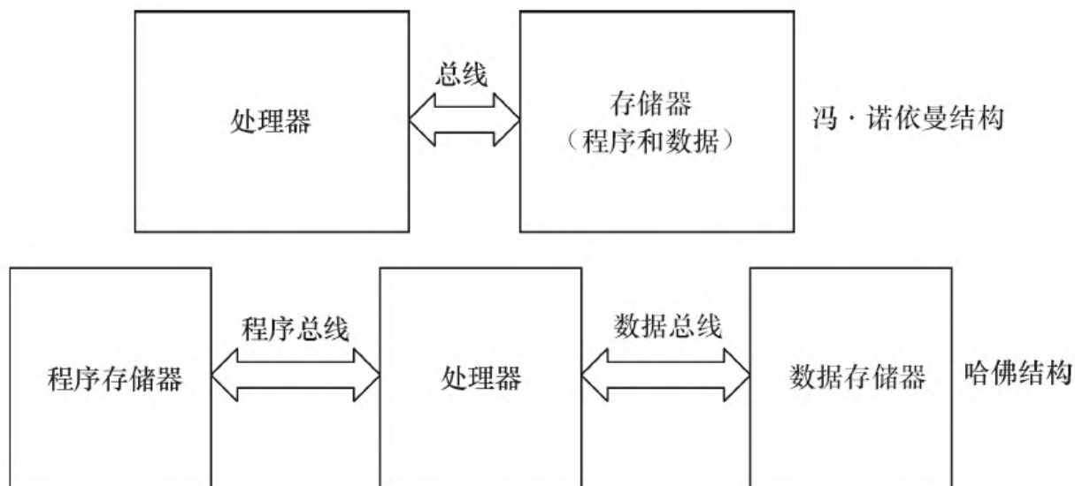
图2.2 冯·诺依曼结构与哈佛结构
