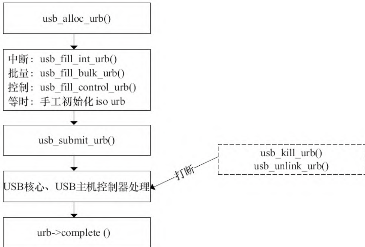
图16.4 URB处理流程
