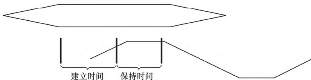
图2.25 建立时间和保持时间
