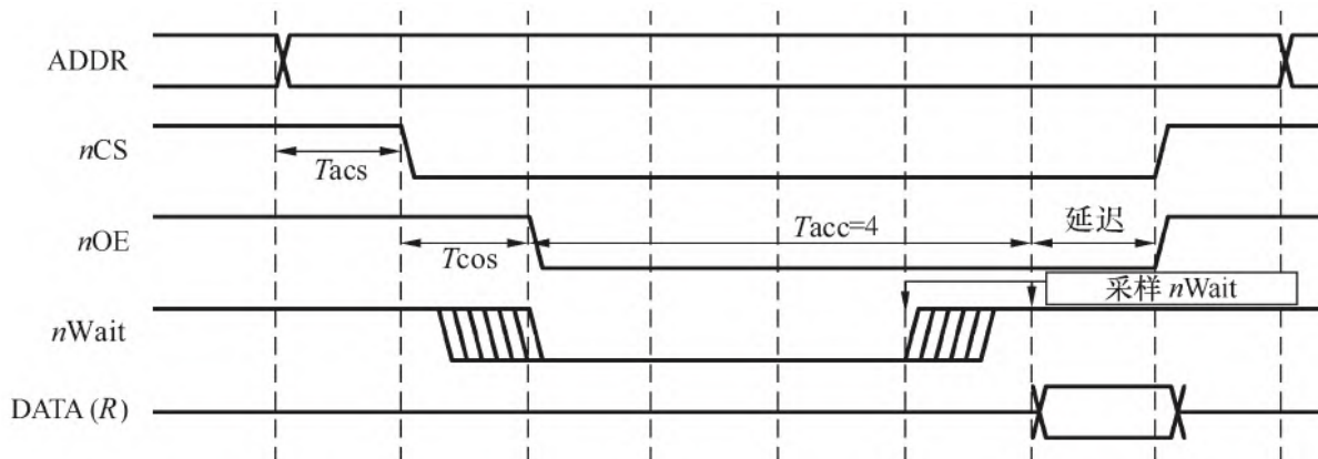
图2.26 SRAM读时序图
