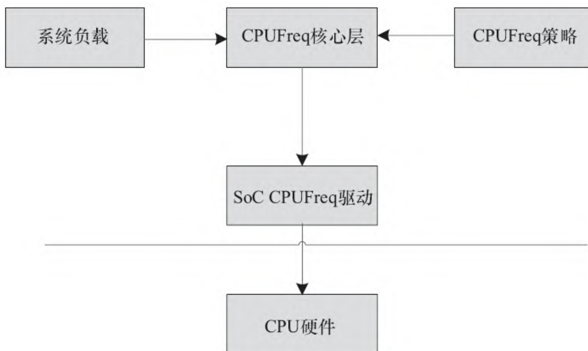
图19.2 CPUFreq、系统负载、策略与调频
