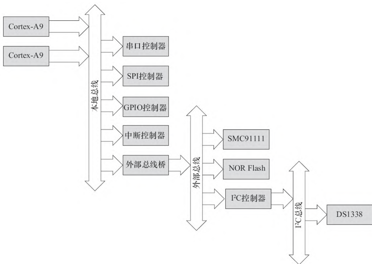
图18.1 设备树参考硬件结构图
