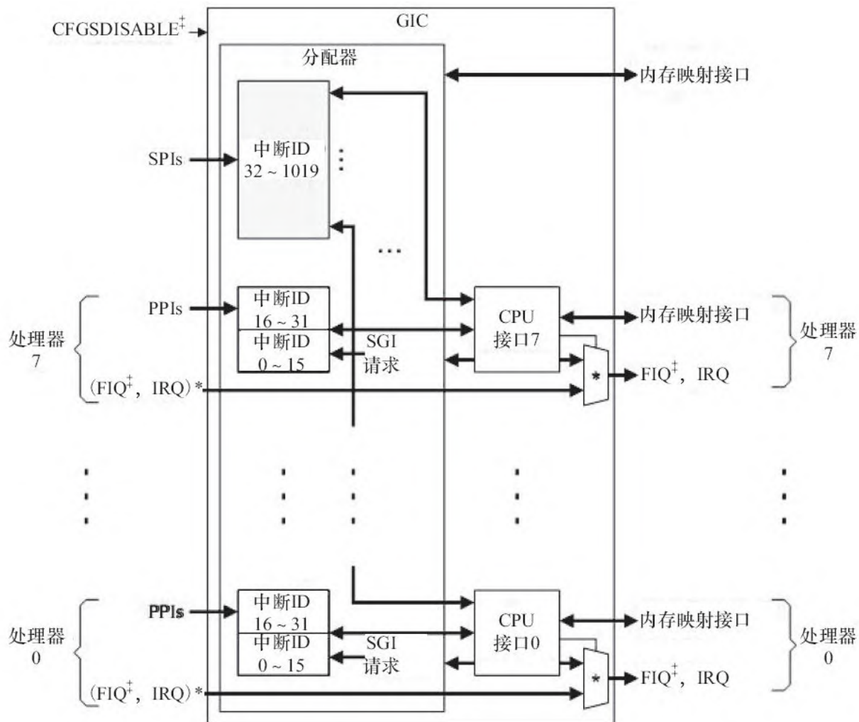
图10.2 ARM多核处理器里的GIC
