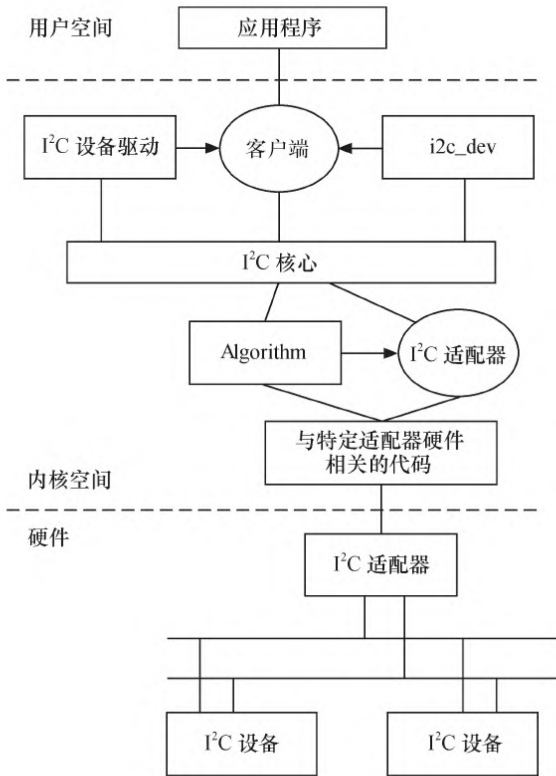
图15.1 Linux的I 2 C体系结构
