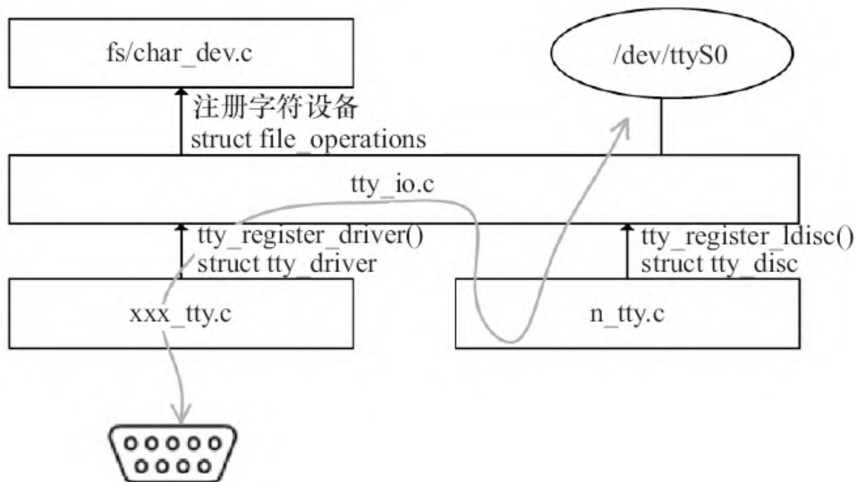
图12.9 Linux内核中tty的层次结构
