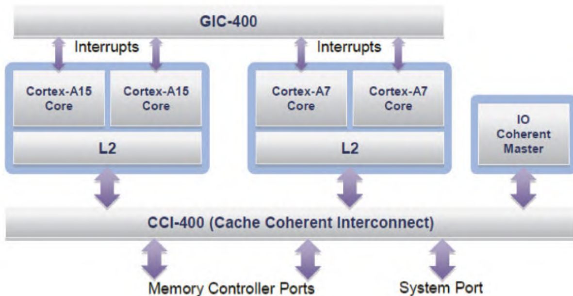
图19.8 ARM的big.LITTLE架构
