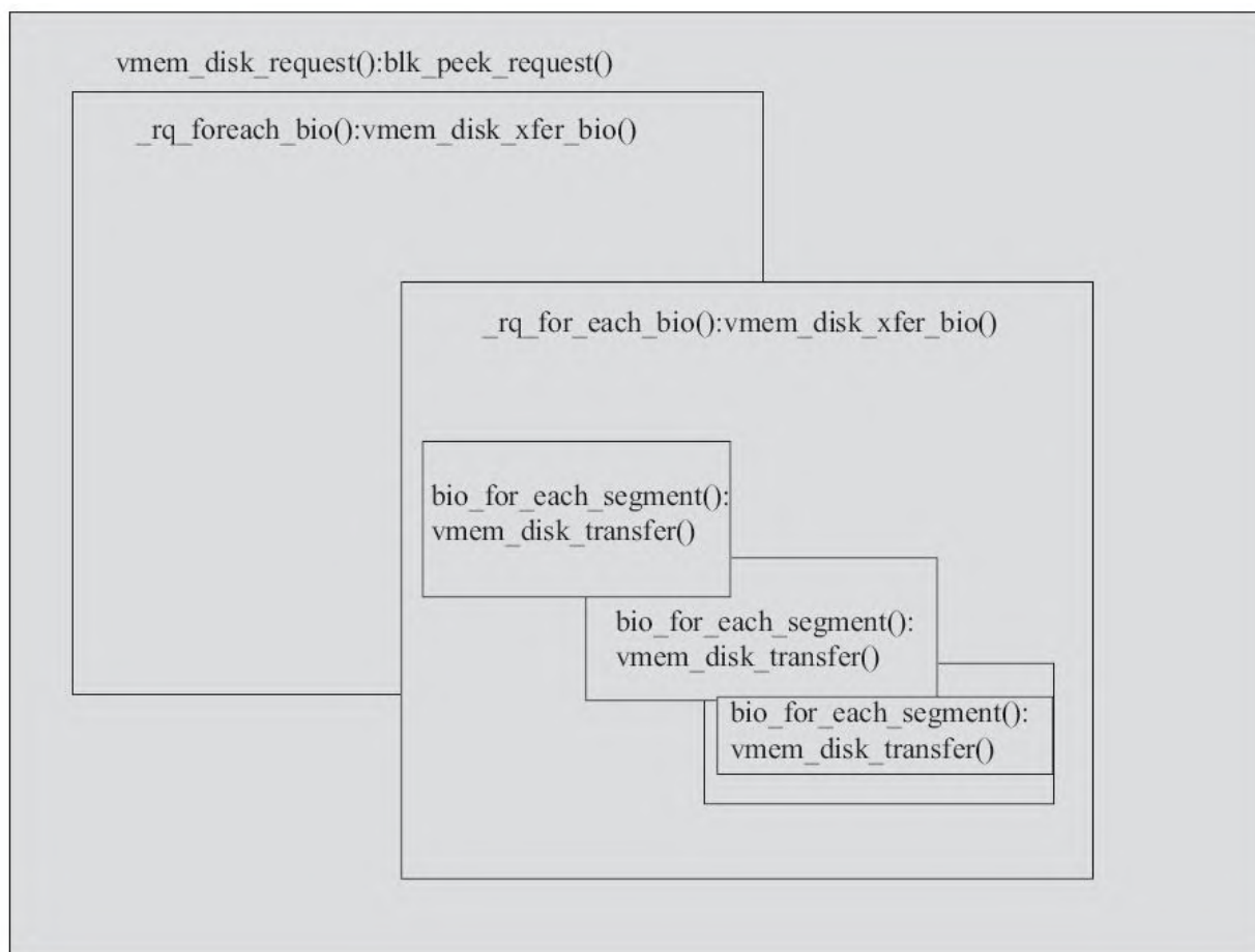
图13.4 vmem_disk的I/O处理过程
