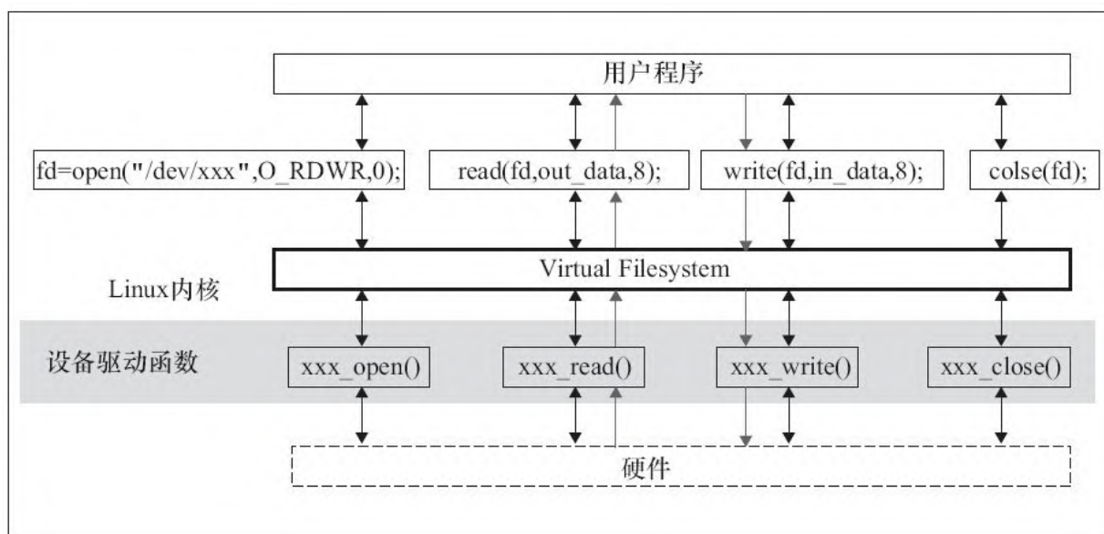
图5.2 应用程序、VFS与设备驱动
