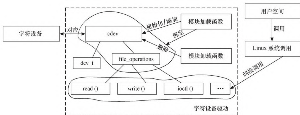
图6.1 字符设备驱动的结构
