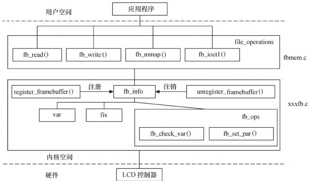
图12.8 Linux帧缓冲设备驱动的程序结构
