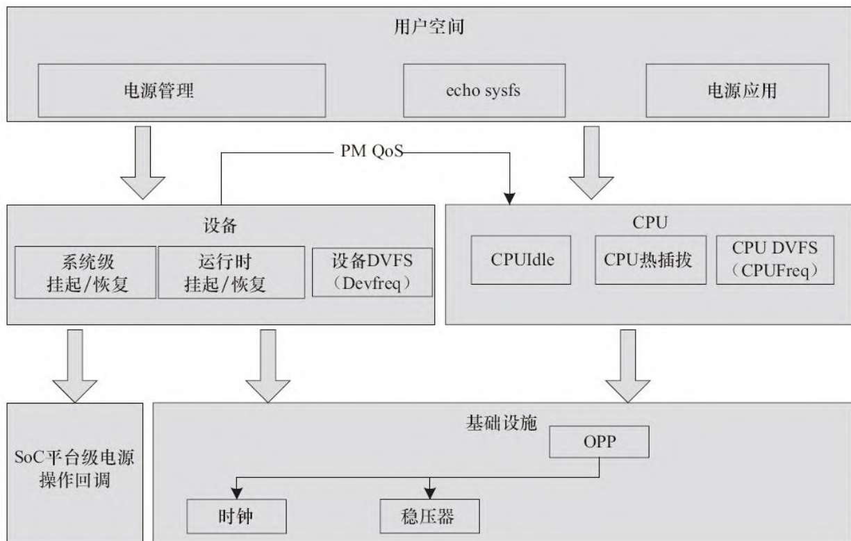
图19.1 Linux内核电源管理的整体架构
