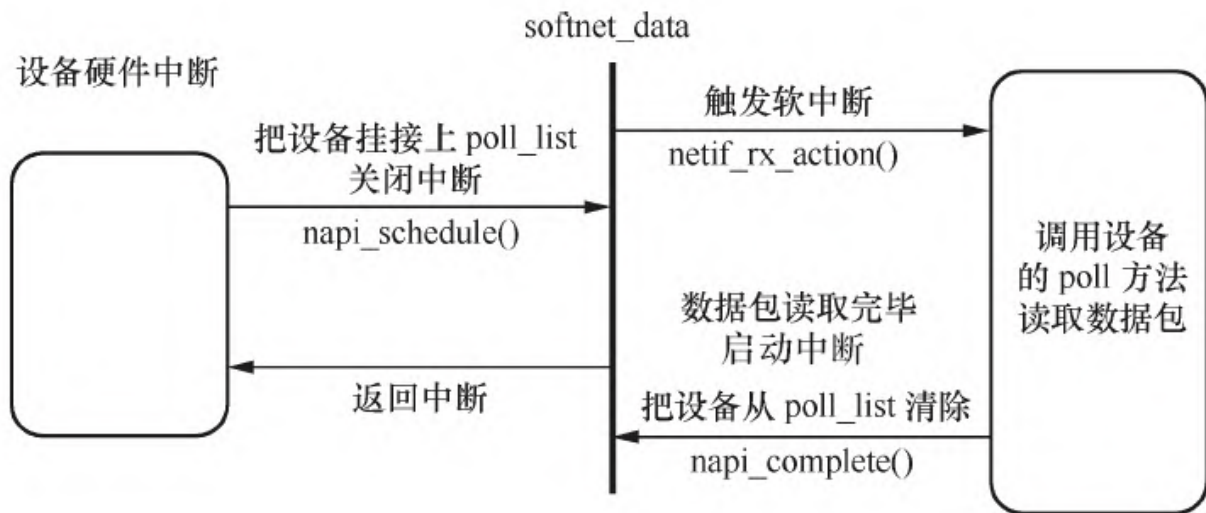
图14.3 NAPI驱动程序各部分的调用关系
