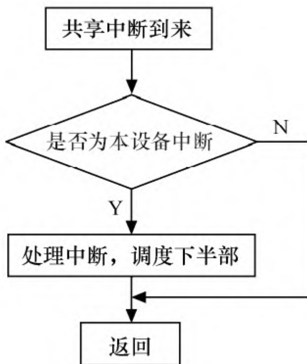
图10.5 共享中断的处理
