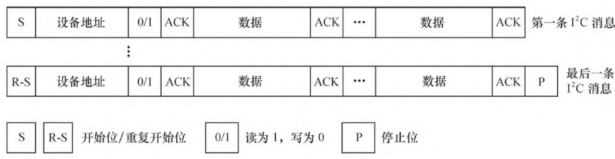
图15.3 master_xfer（）完成的时序
