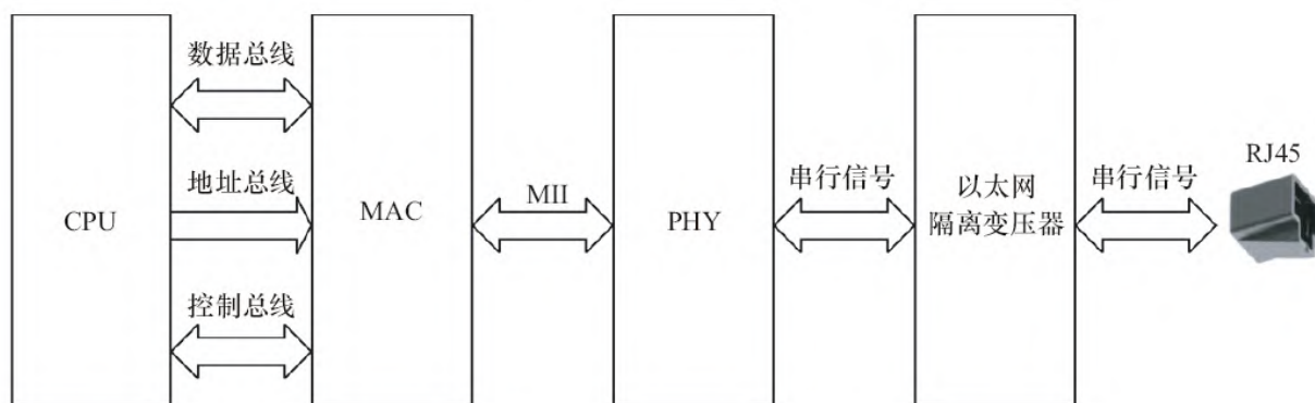
图2.15 以太网接口的硬件电路原理
