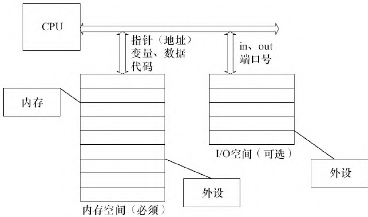
图11.1 内存空间和I/O空间
