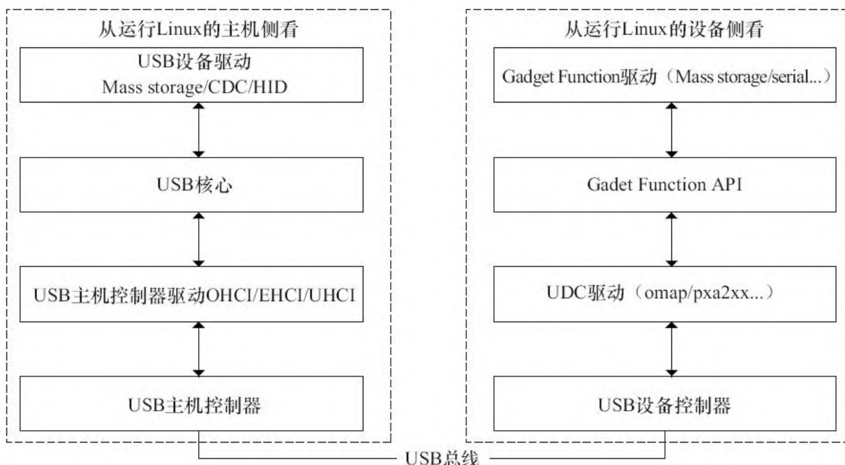
图16.1 Linux USB驱动总体结构
