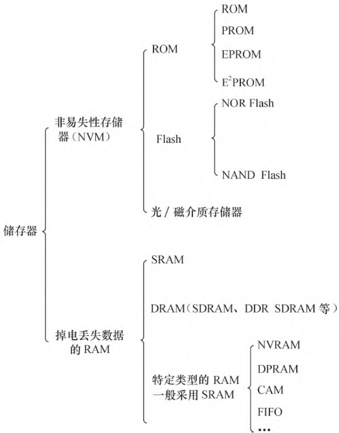
图2.8 存储器分类
