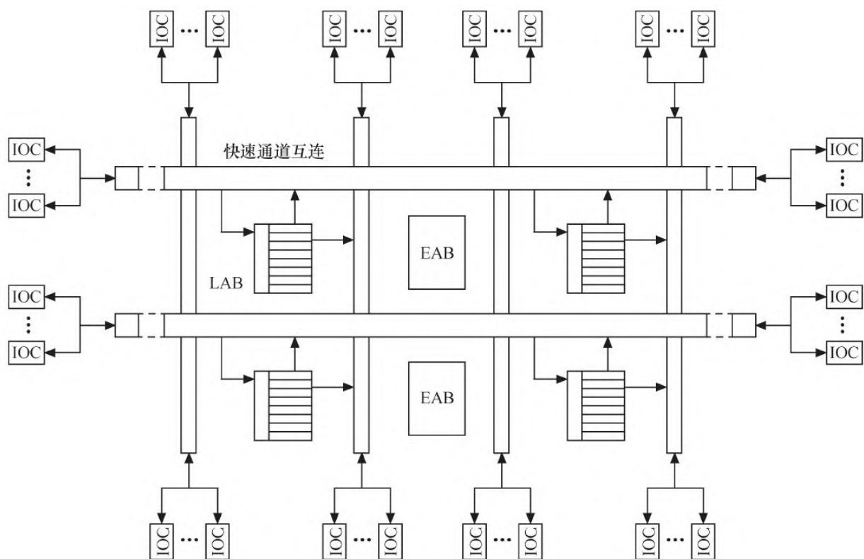
图2.21 典型的FPGA内部结构
