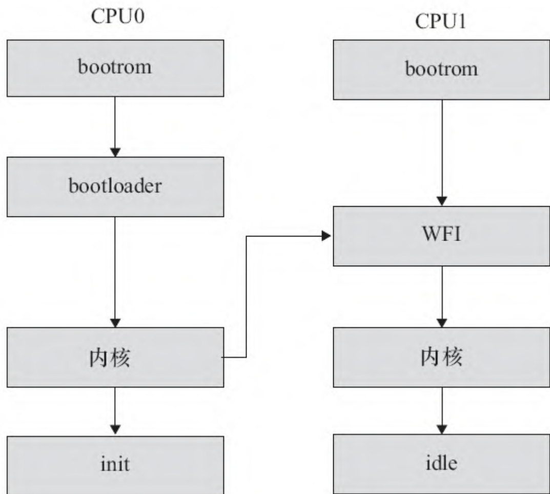
图3.11 ARM上的Linux引导流程
