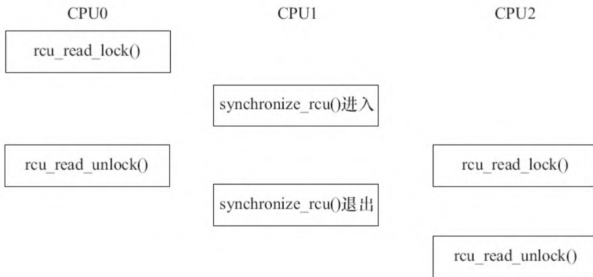
图7.9 synchronize_rcu
