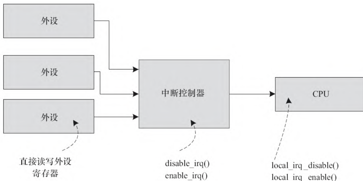
图20.3 屏蔽中断的3个不同位置
