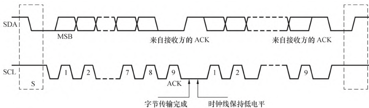
图2.11 I 2 C总线的时序
