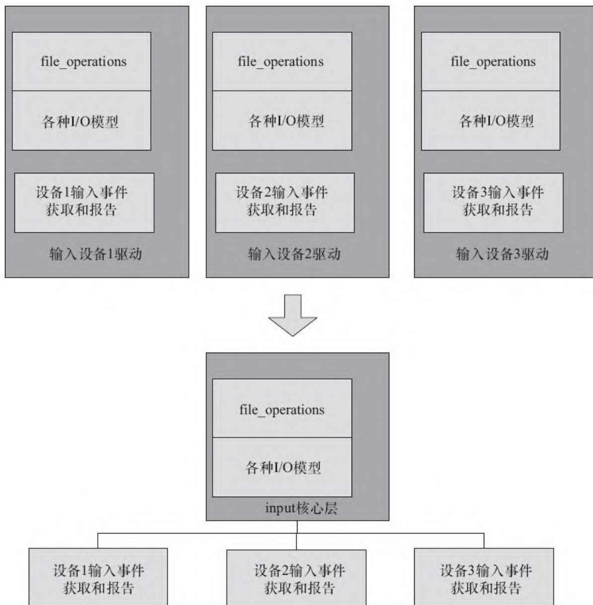
图12.2 Linux驱动的分层
