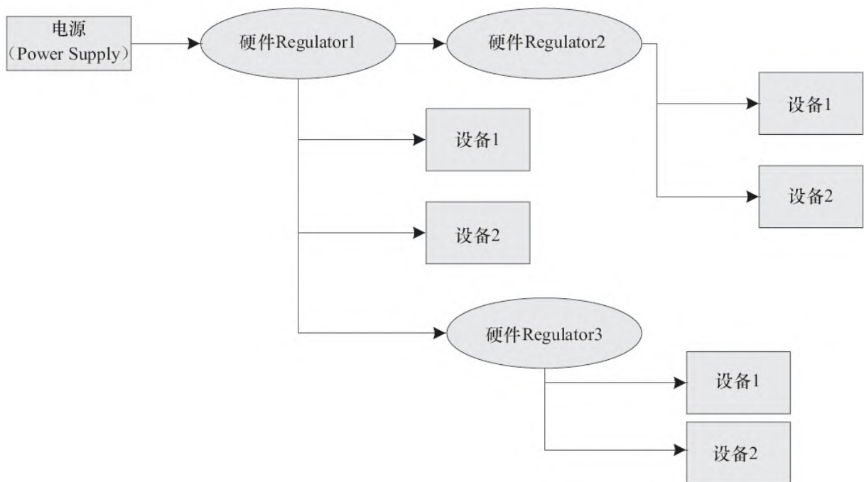
图19.6 Regulator树形结构
