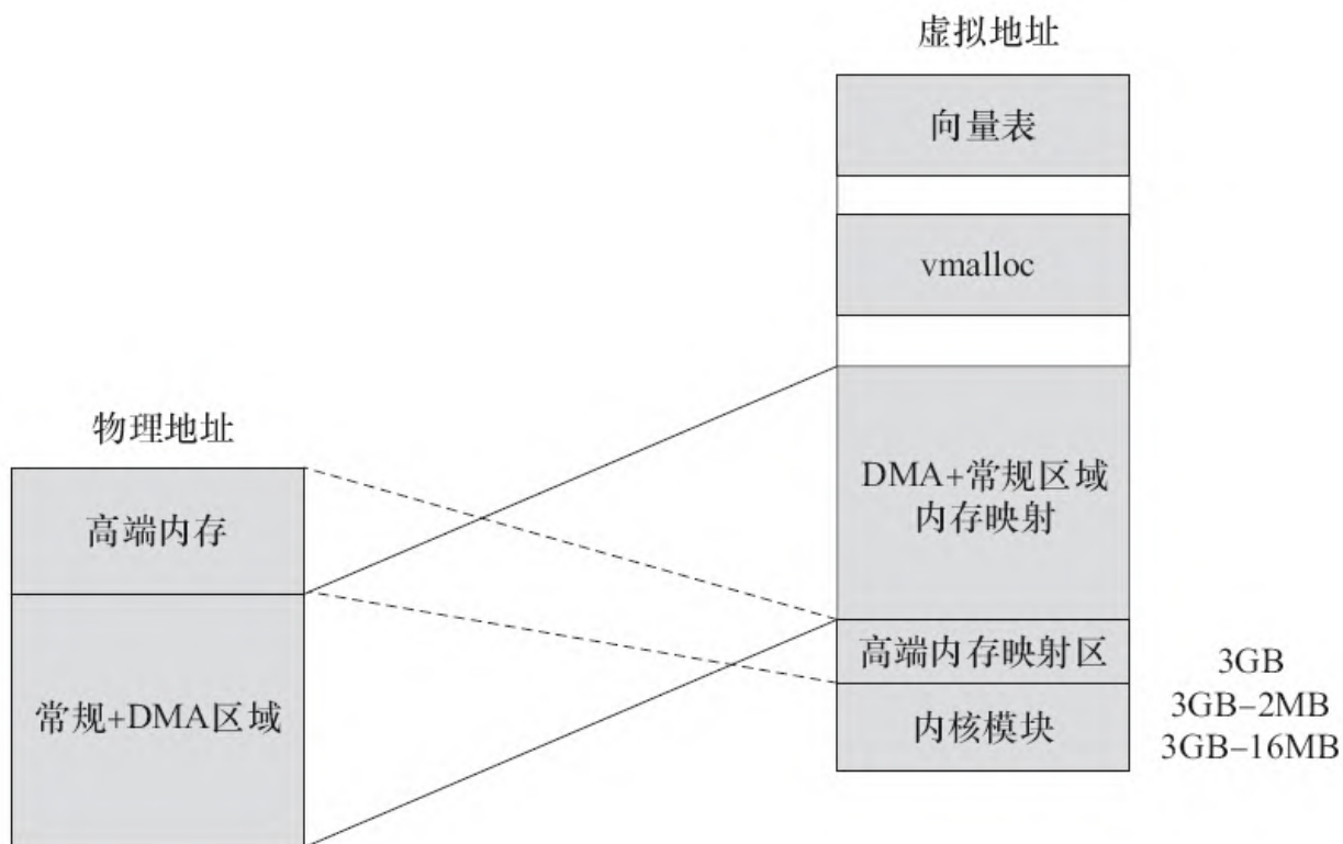
图11.7 32位ARM系统中Linux内核的地址空间
