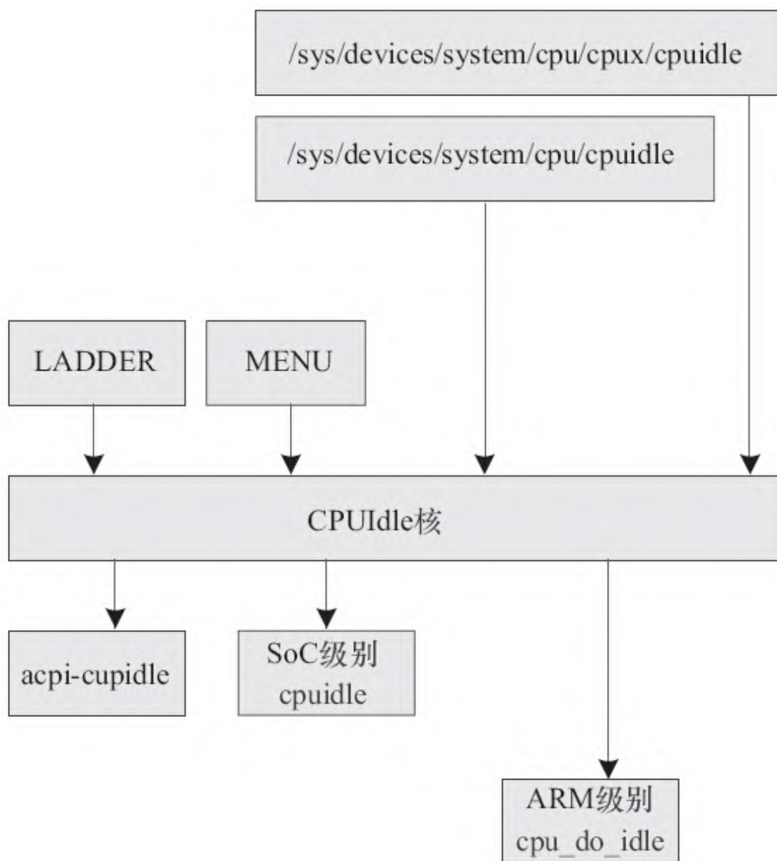
图19.4 Linux CPUIIdle子系统的整体架构
