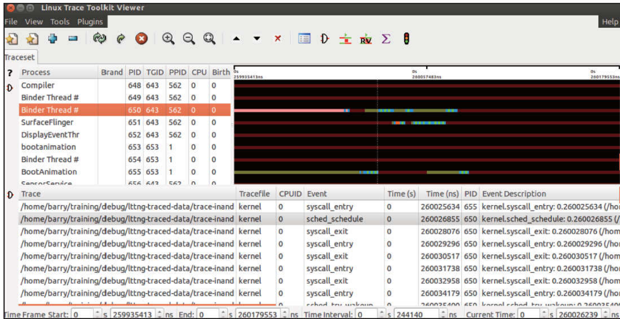
图21.9 LTTng形成的时序图
