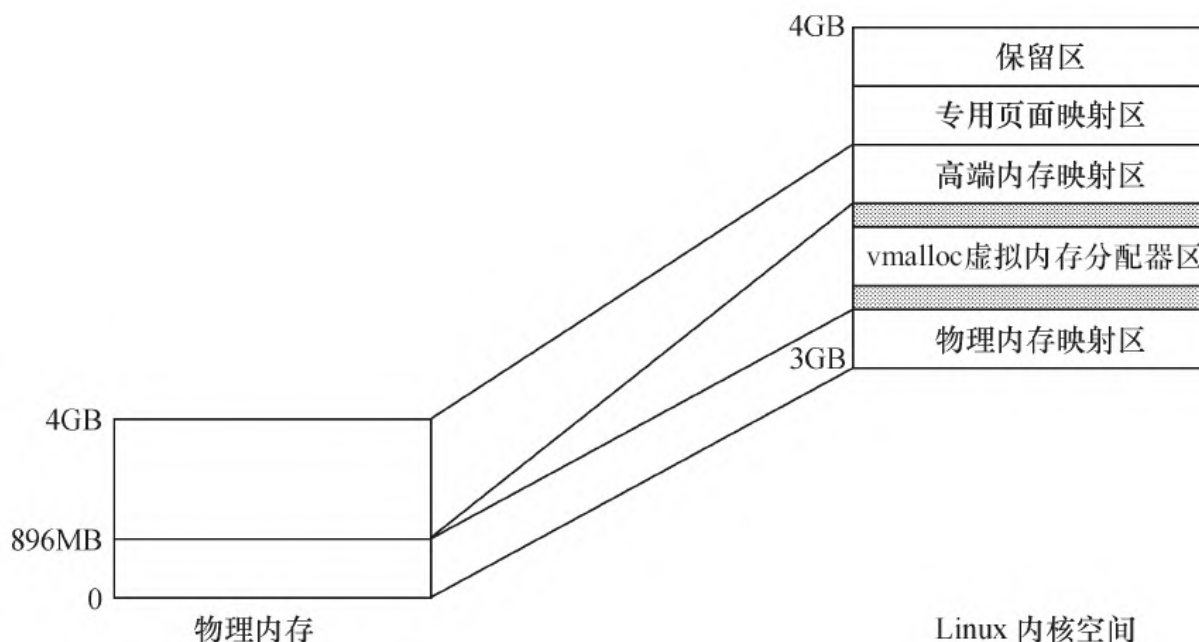
图11.6 32位x86系统Linux内核的地址空间
