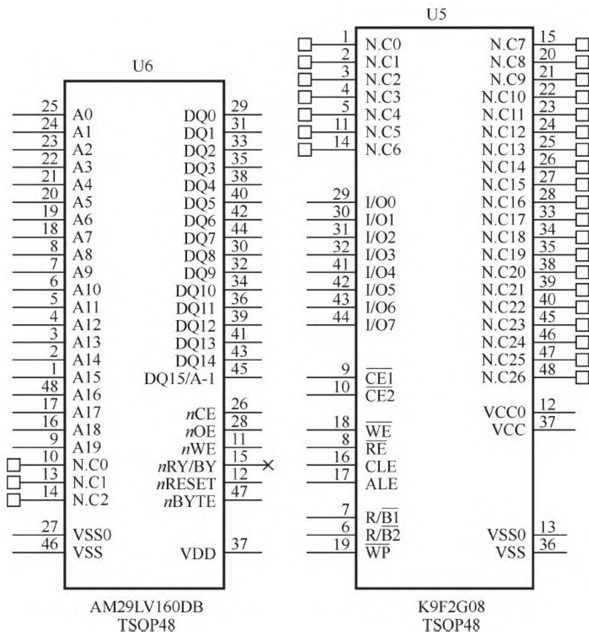
图2.22 原理图中的符号
