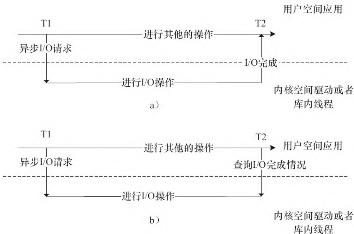
图9.3 异步I/O的时序
