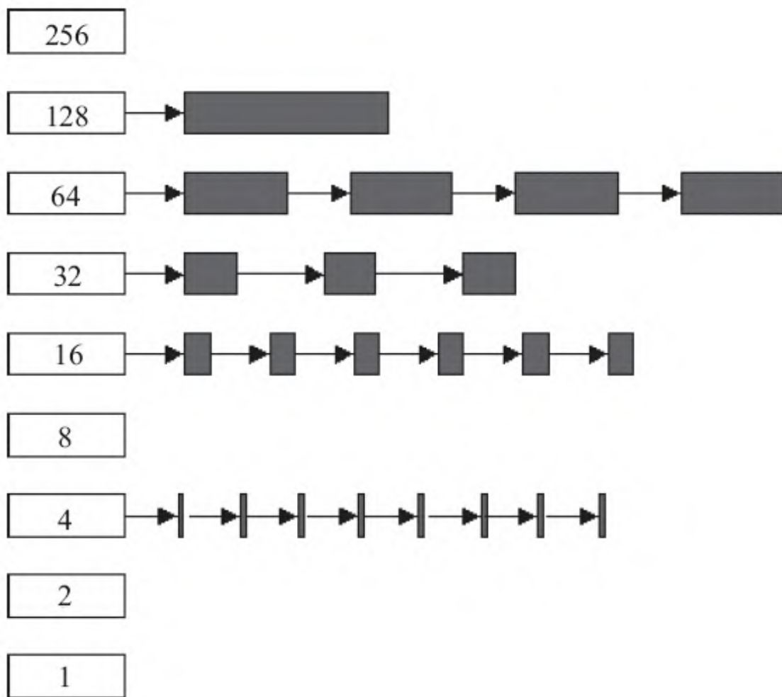
图11.9 buddy算法
