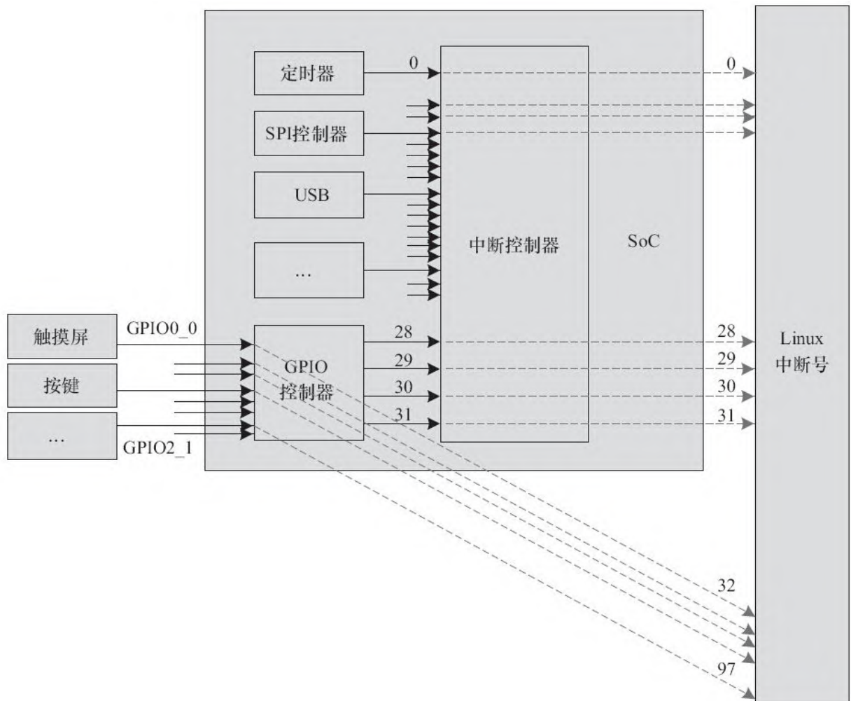
图20.5 中断级联与映射
