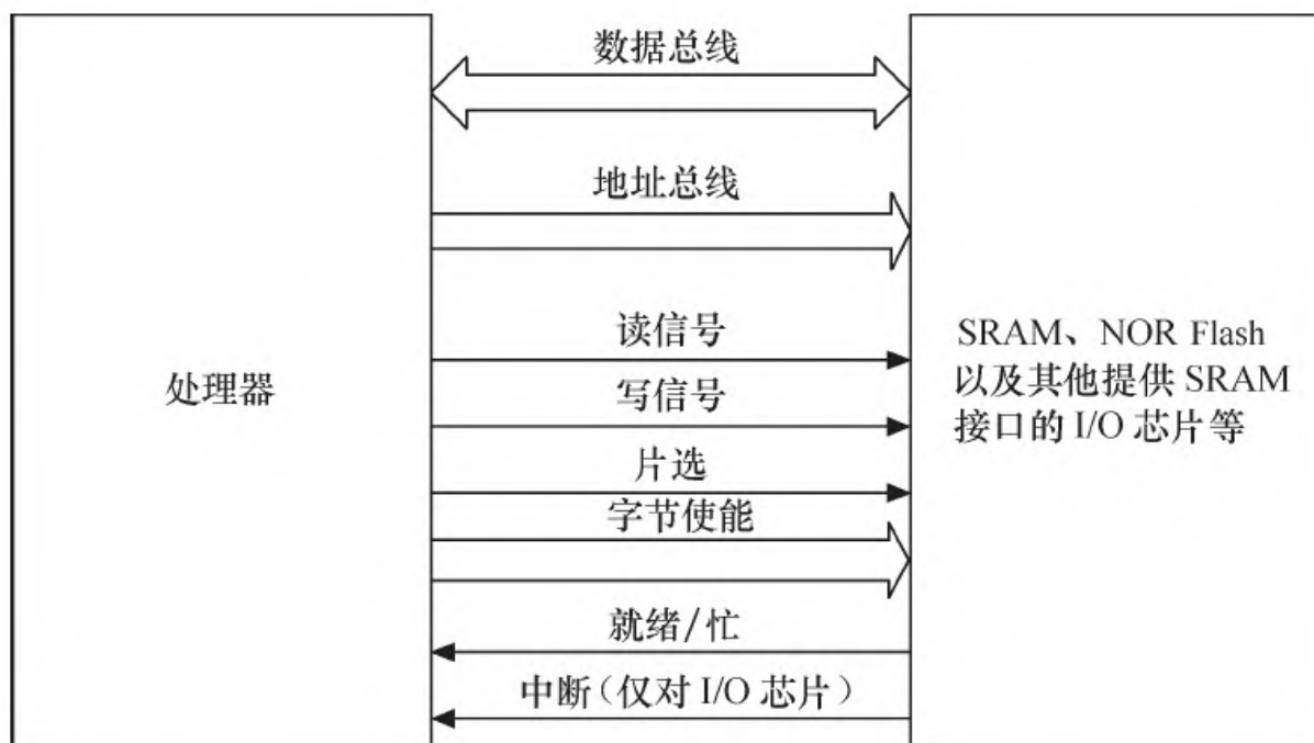
图2.5 典型的类SRAM接口
