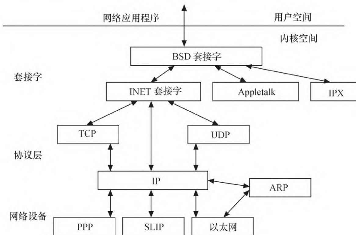
图3.8 Linux网络体系结构
