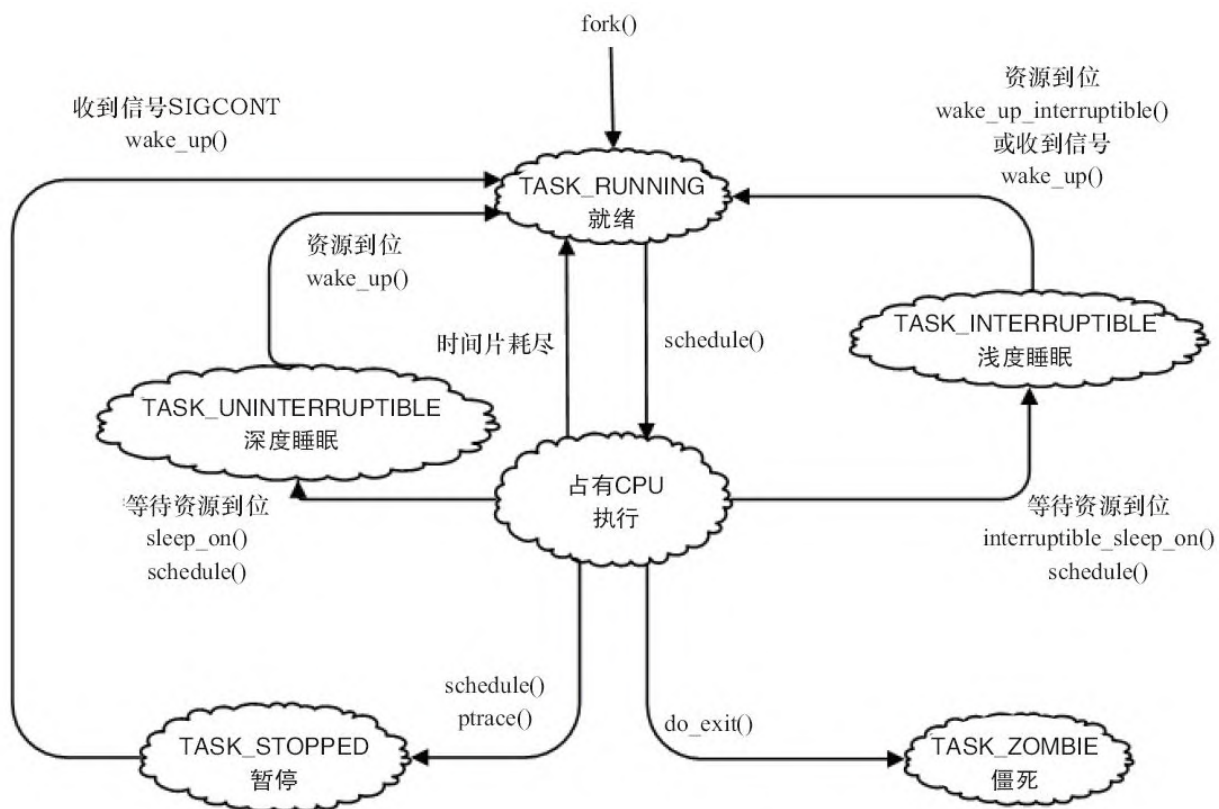
图3.4 Linux进程状态转换
