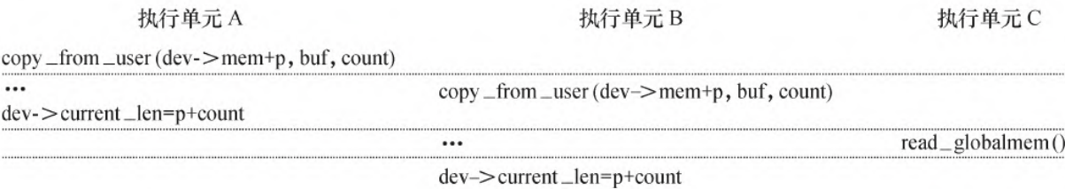
图7.2 并发执行单元的交错执行
