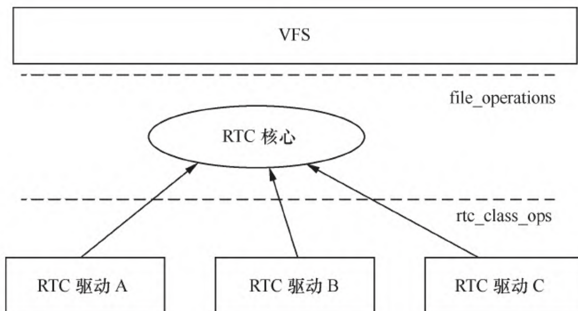
图12.7 Linux RTC设备驱动的分层
