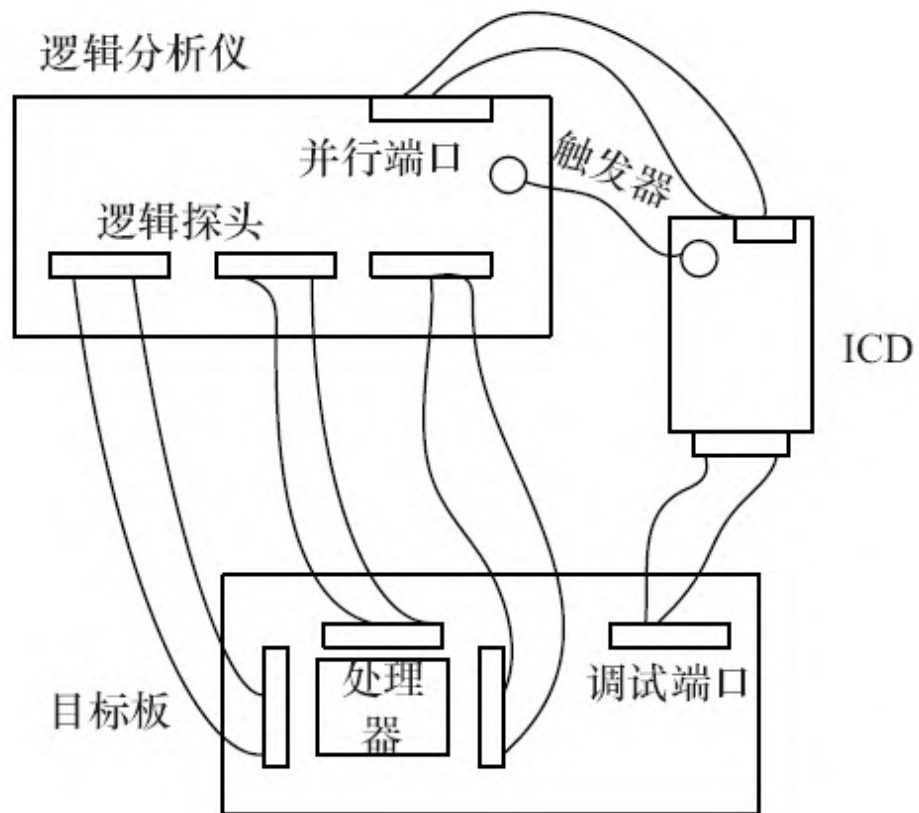
图2.35 逻辑分析仪与ICD协作
