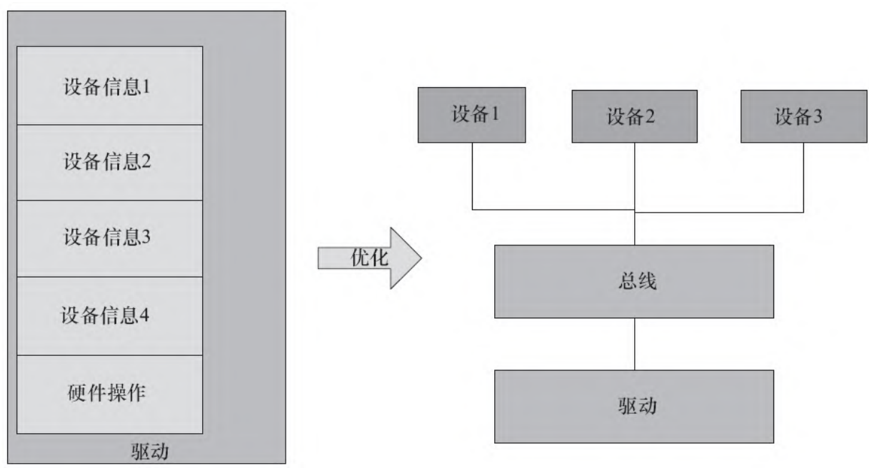
图12.1 Linux设备和驱动的分离
