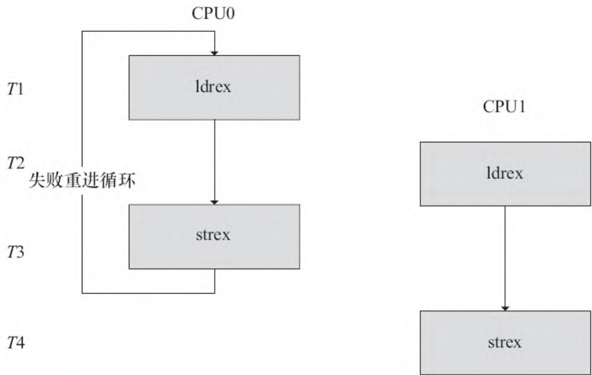
图7.6 ldrex和strex指令
