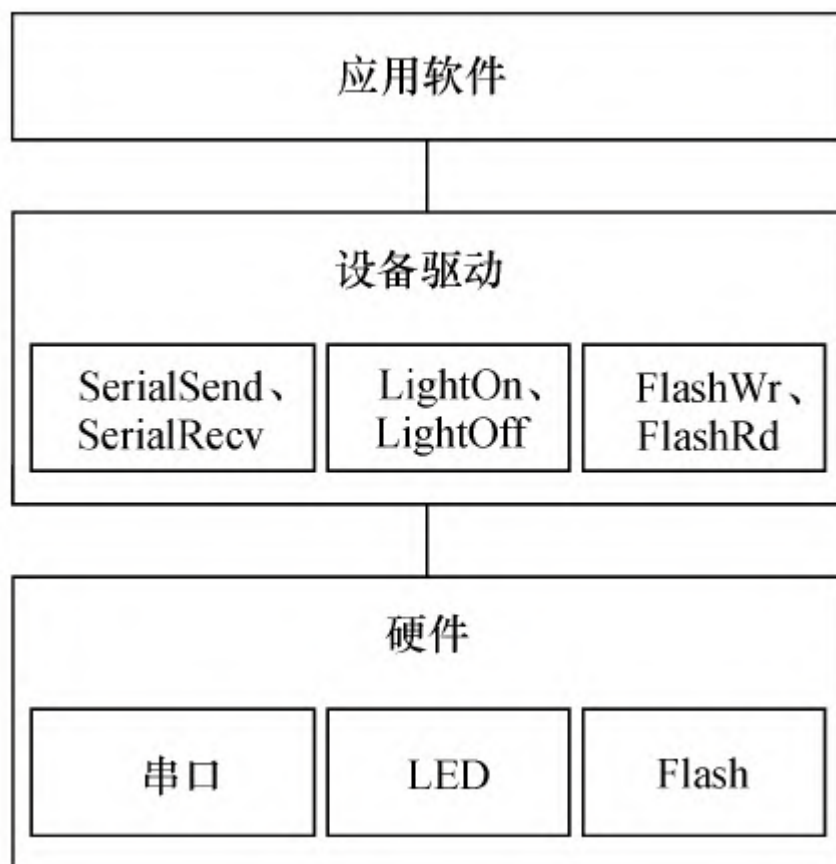
图1.1 无操作系统时硬件、设备驱动和应用软件的关系
