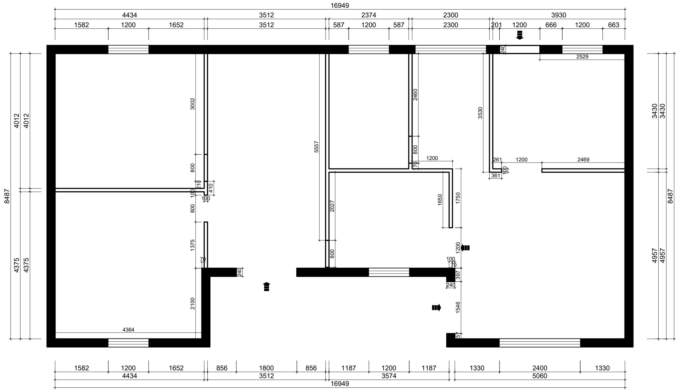
墙体定位(1:65)
