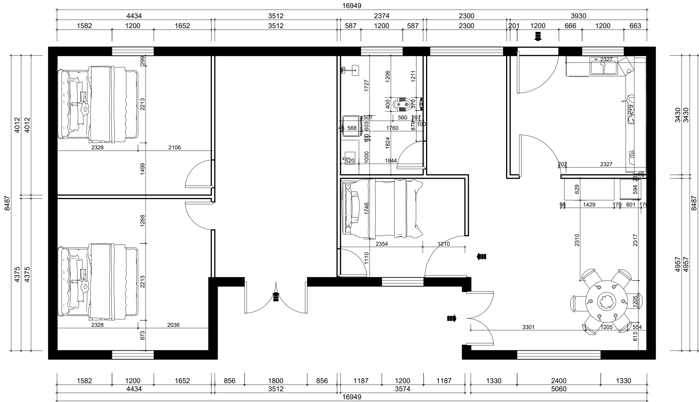
家具尺寸(1:65)
