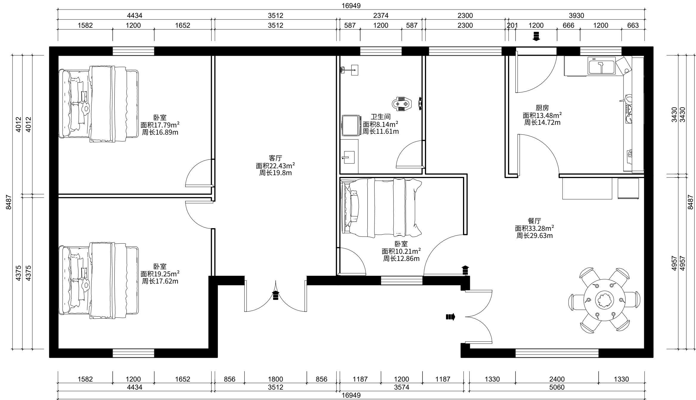
平面布置(1:65)
