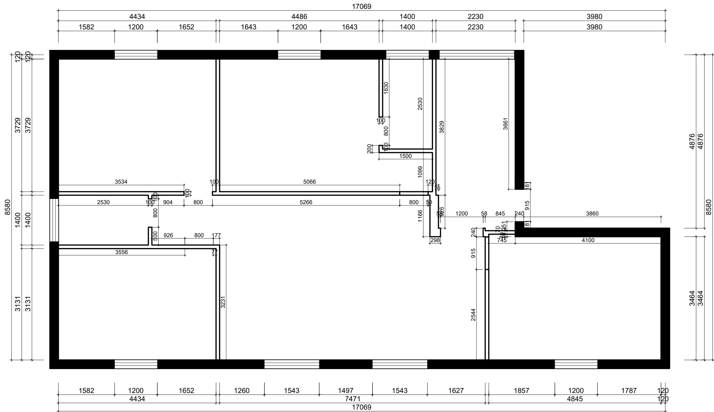
墙体定位(1:65)
