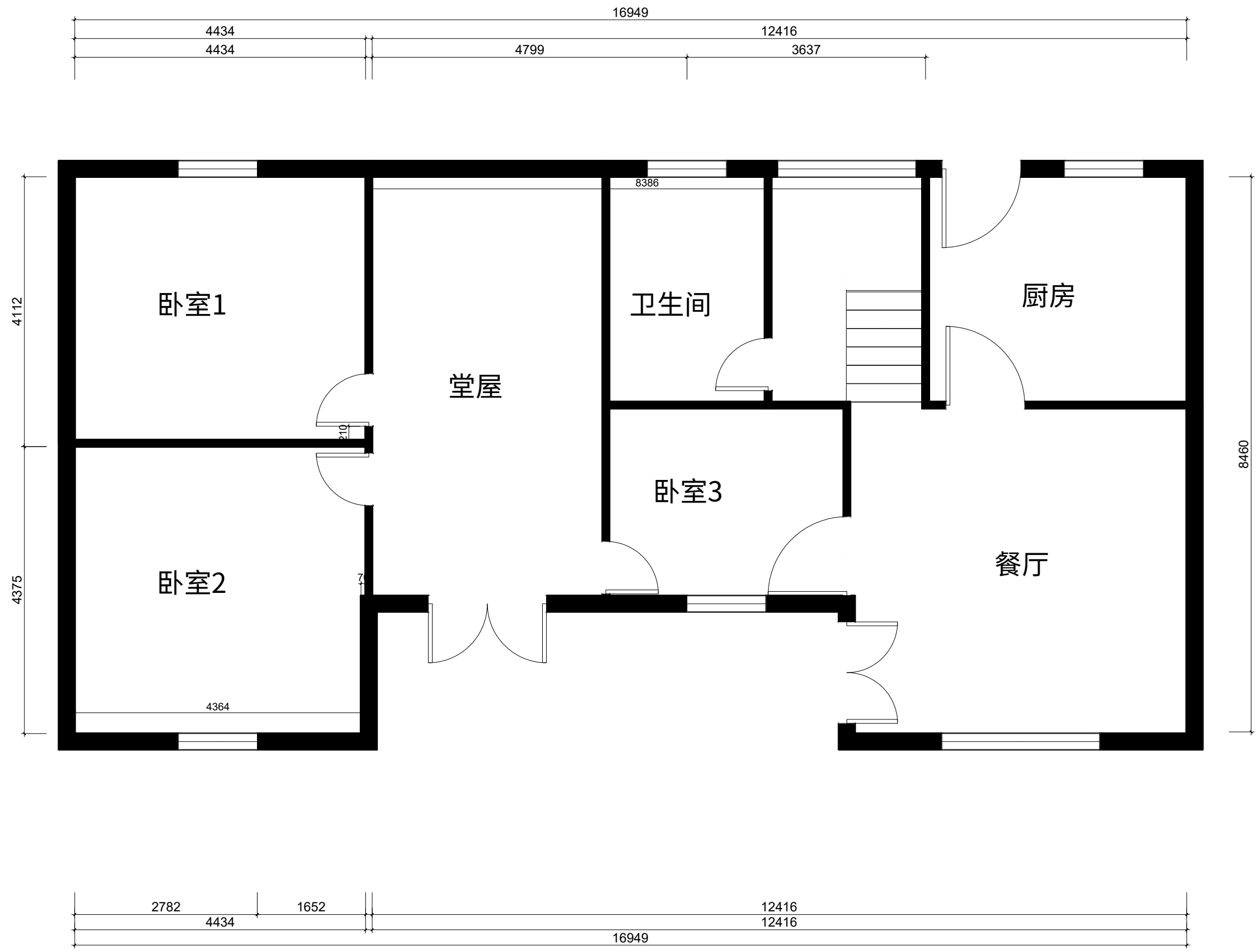
楼层1平面(1:65)
