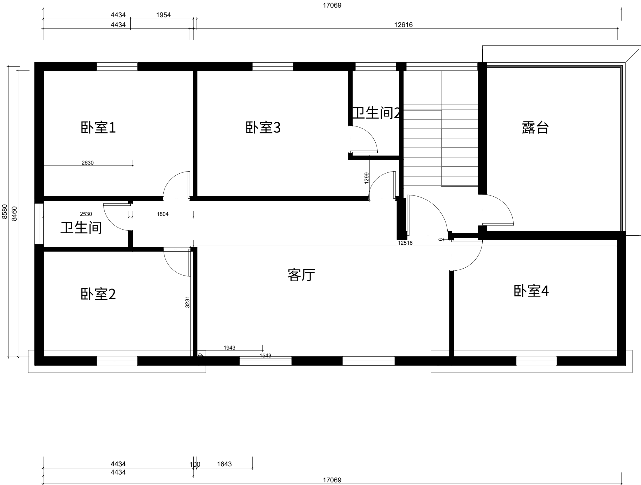
楼层2平面(1:65)
