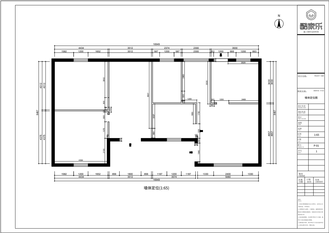
图 1: 一楼设计图
