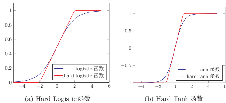
图 4.3 Hard Sigmoid 型激活函数
