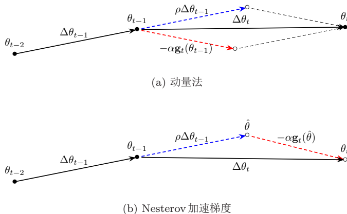
图 7.6 动量法和 Nesterov 加速梯度的比较
