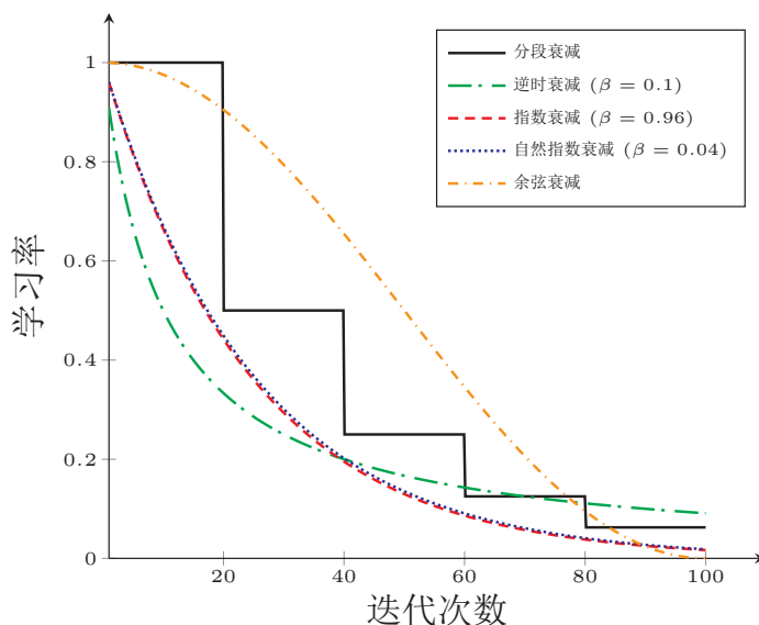
图 7.4 不同学习率衰减方法的比较
