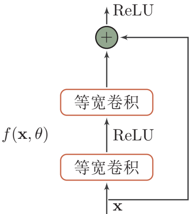
图 5.15 一个简单的残差单元结构
