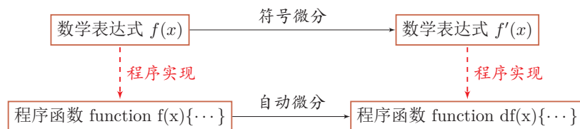
图 4.9 符号微分与自动微分对比
