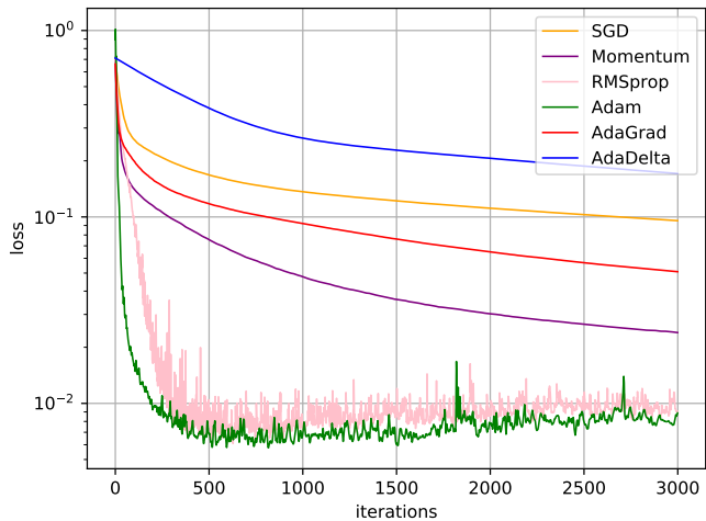
图 7.8 不同优化方法的比较
