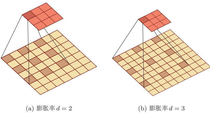
图 5.18 空洞卷积
