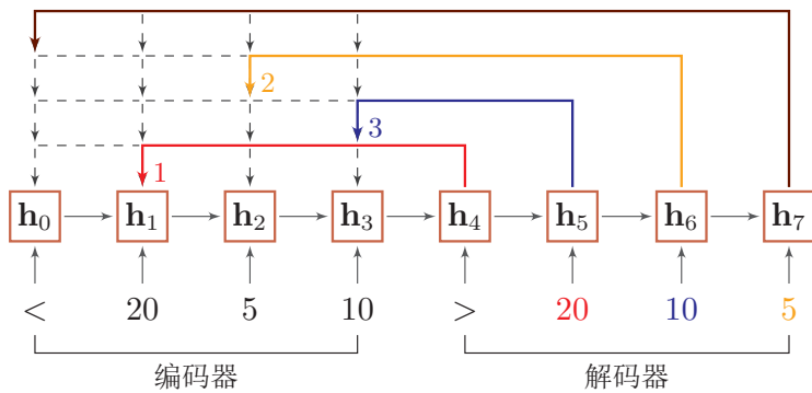
图 8.2 指针网络
