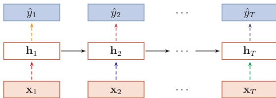
图 7.13 针对非循环连接的丢弃法
