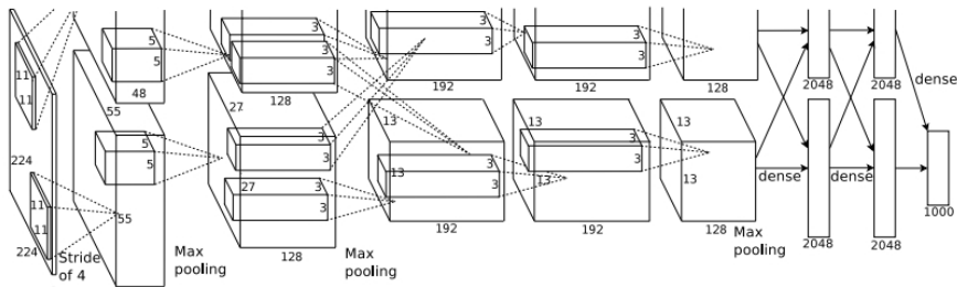
图 5.12 AlexNet 网络结构(图片来源于 [Krizhevsky et al., 2012])
