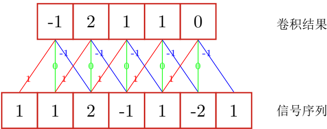
图 5.1 一维卷积示例(滤波器为[-1, 0, 1])
