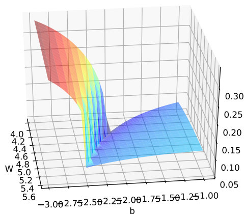
图 7.7 梯度爆炸问题示例
