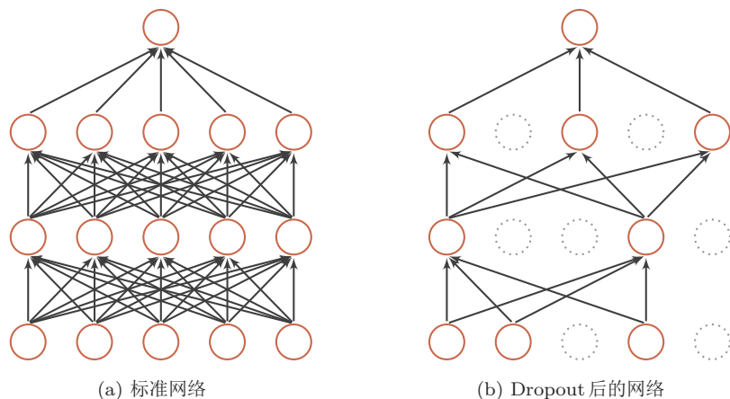
图 7.12 丢弃法示例
