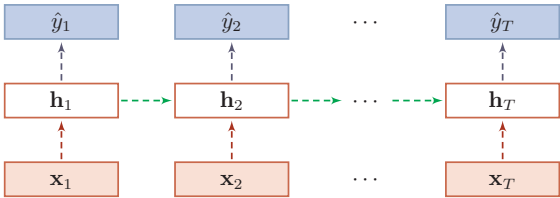
图 7.14 变分丢弃法
