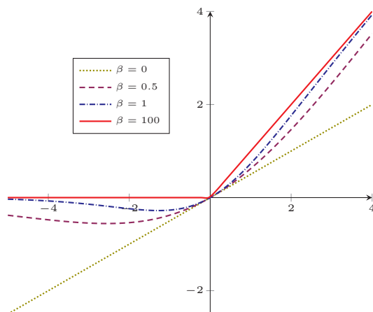
图 4.5 Swish 函数
