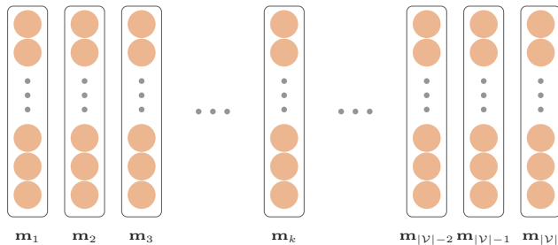
图 15.2 嵌入矩阵
