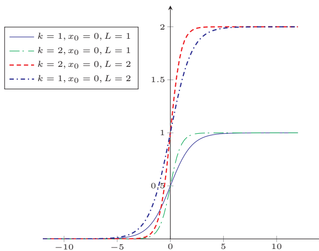
图 B.2 Logistic 函数
