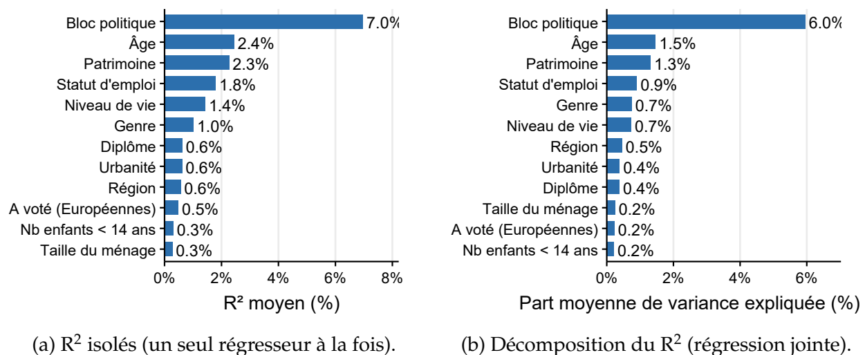
Figure A1: Variance dans les attitudes expliquée par les caractéristiques sociodémographiques. (a) R^2 moyen obtenu en régressant chaque attitude sur une seule caractéristique à la fois ; (b) part moyenne de variance expliquée par chaque caractéristique dans la régression jointe (décomposition LMG, variance expliquée totale : 13 %). Les moyennes sont calculées sur les 49 variables d'attitudes (mesures budget, programme et indices somme_convenable et somme_souhaitable).
