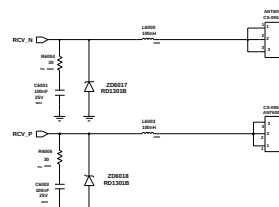
RCV CONTACT
