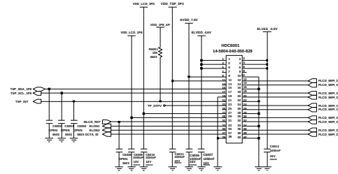
5.5" HD OCTA CON
