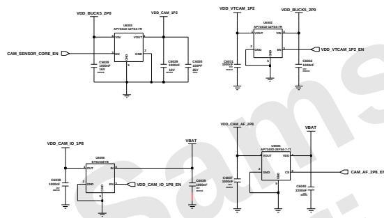
13M CAMERA CON
