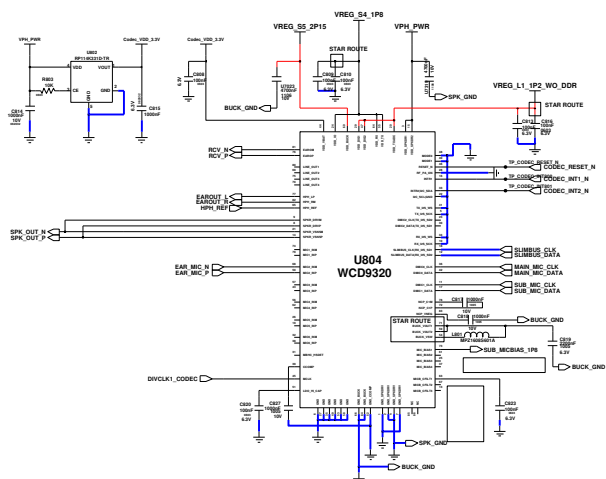
Audio Codec
