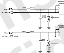
RCV CONTACT
