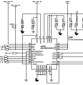
RCV AMP
