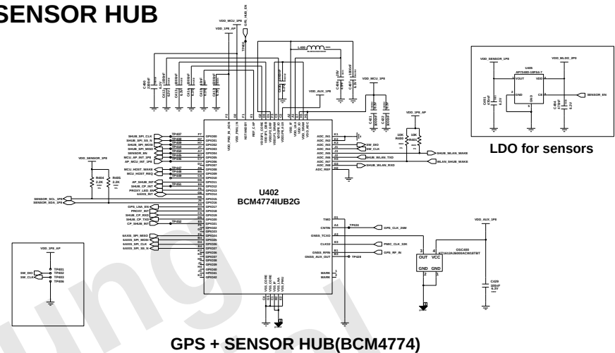
GPS + SENSOR HUB(BCM4774)
