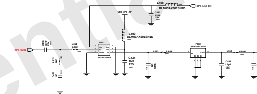
GPS + SENSOR HUB(BCM4774)
