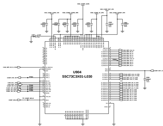
COMPANION IC
