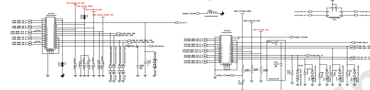
MAIN_CAMERA (13M) : SM-J330F
