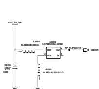
Hall IC
