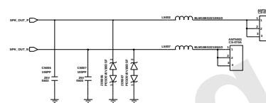
SPK CON
