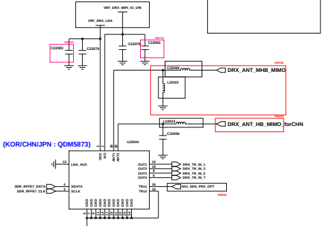
DRX_MHB_2 (B2/4/7/25/30/41/66)
