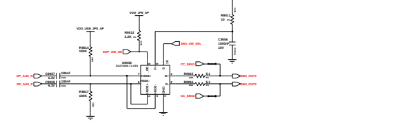
AUX SW
