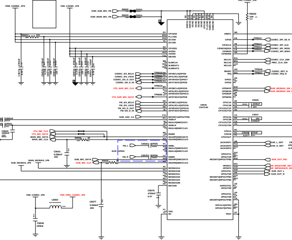
AUDIO CODEC
