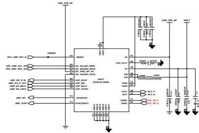
RCV AMP
