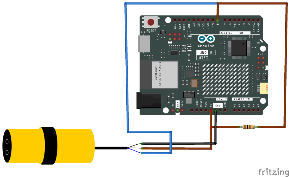
Figure 4.4.: Anschluss der Lichtschanke an einen Mikokontroller mit einem Pull-up-Widerstand ( R = 10K\Omega )
