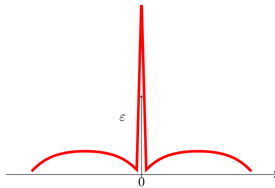
Abbildung 23.5.: Abweichung bei Vorgabe des Abstands L bei der Verrundung mit einem Kreisbogen
