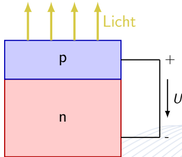
Abbildung: Funktionsprinzip einer LED [JW14]
