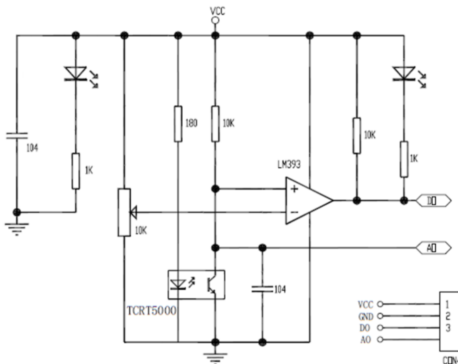
Figure 4.3.: Beispielhafte Darstellung der Schaltung einer Infrarot-Lichtschranke anhand des Moduls TCRT5000 IR [Lip18], ein Modul ähnlich dem der E18-D80NK
