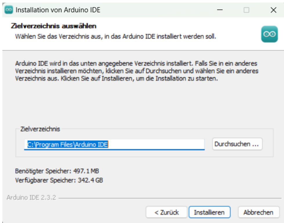
Abbildung 5.4.: Zielverzeichnisauswahl
