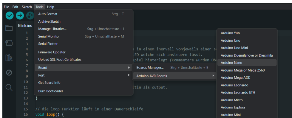
Abbildung 5.5.: Boardauswahl
