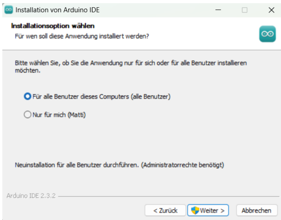
Abbildung 5.3.: Installationsoption
