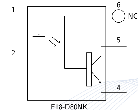
Abbildung: Schaltplan des E18-D80NK
