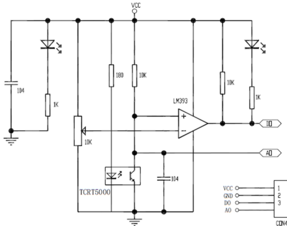
Abbildung 4.3.: Beispielhafte Darstellung der Schaltung einer Infrarot-Lichtschranke anhand des Moduls TCRT5000 IR [Hes09], ein Modul ähnlich dem der E18-D80NK
