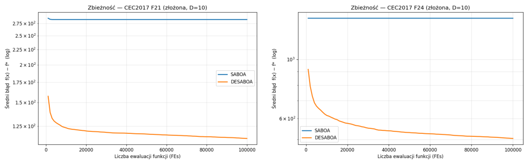
Rysunek 5: Krzywe zbienoci – CEC2017 F21 oraz F24 (D=10).
