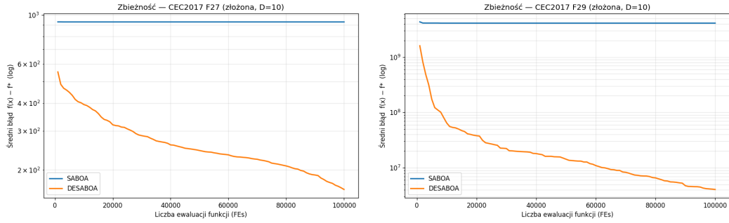
Rysunek 6: Krzywe zbienoci – CEC2017 F27 oraz F29 (D=10).
