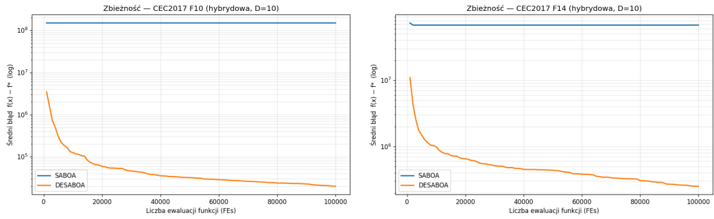
Rysunek 3: Krzywe zbienoci – CEC2017 F10 oraz F14 (D=10).
