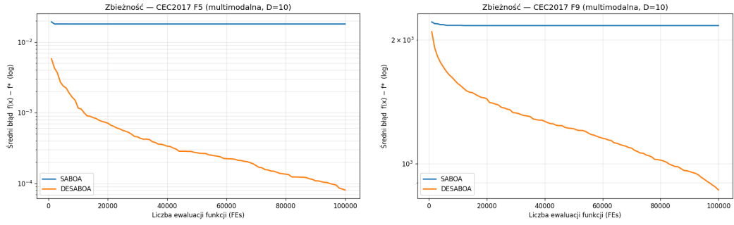
Rysunek 2: Krzywe zbienoci – CEC2017 F5 oraz F9 (D=10).
