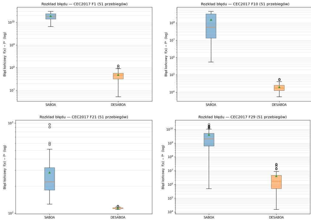
Rysunek 7: Rozkady bdu kocowego: F1 (unimodalna), F10 (hybrydowa), F21 i F29 (zoone).
