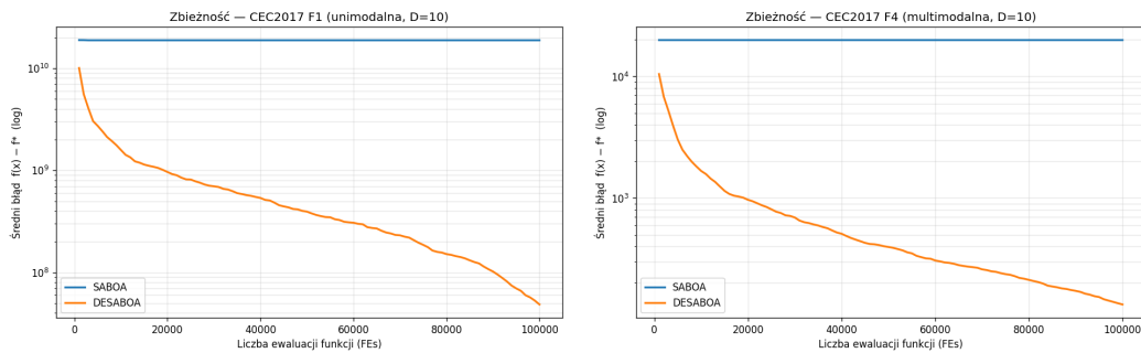
Rysunek 1: Krzywe zbienoci – CEC2017 F1 oraz F4 (D=10).
