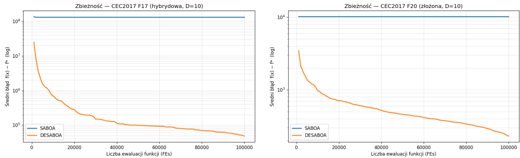
Rysunek 4: Krzywe zbienoci – CEC2017 F17 oraz F20 (D=10).
