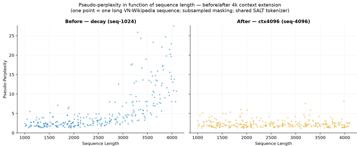
Hình 4.5: Pseudo-perplexity theo độ dài chuỗi trước (trái) và sau (phải) pha mở rộng ngữ cảnh 4.096 token.
