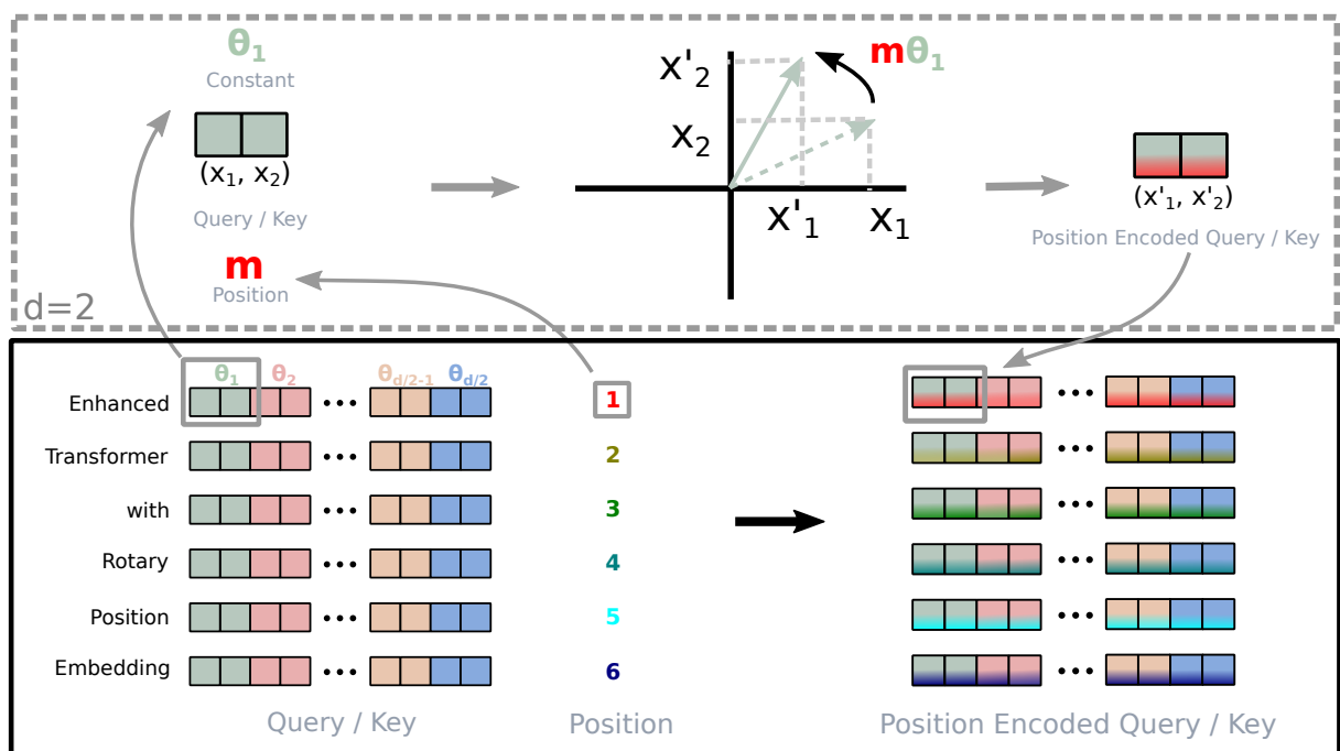
Hình 2.3: Minh họa cơ chế RoPE: mỗi véc-tơ truy vấn/ khóa được quay một góc tỷ lệ với vị trí token, với tần số khác nhau theo từng cặp chiều (Nguồn: Su và cộng sự [13]).
