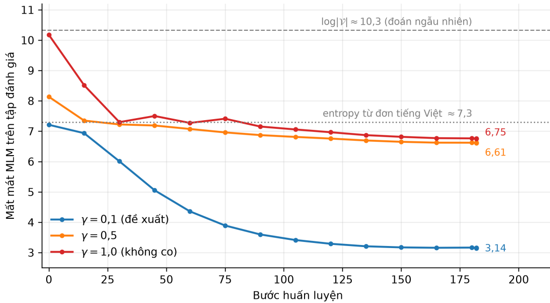
Hình 4.2: Mất mát MLM trên tập đánh giá của ba giá trị hệ số \gamma .
