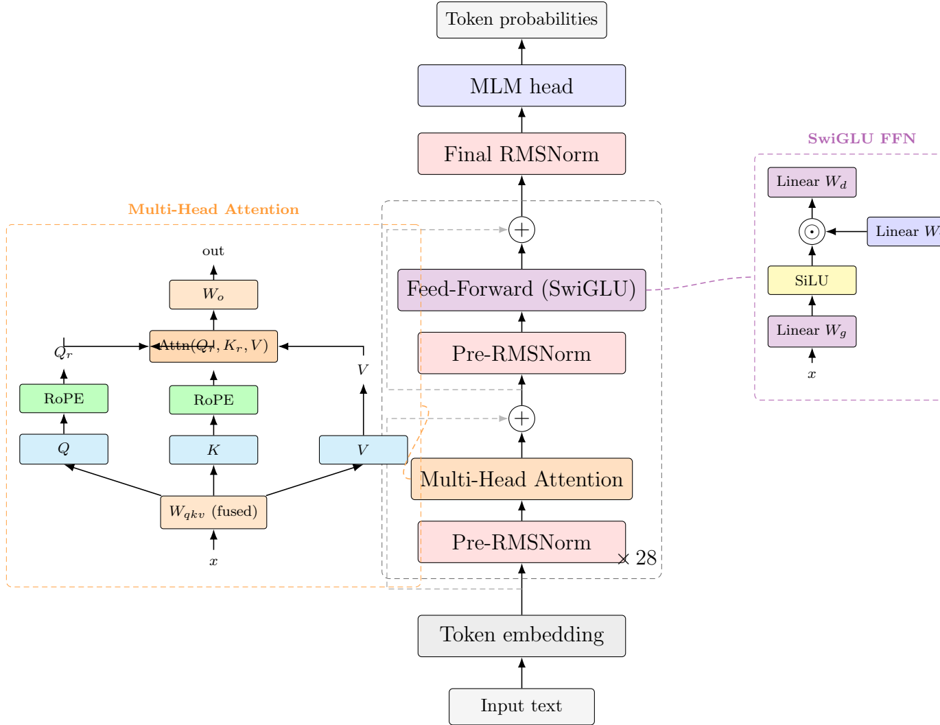
Hình 2.2: Kiến trúc NeoBERT [5].
