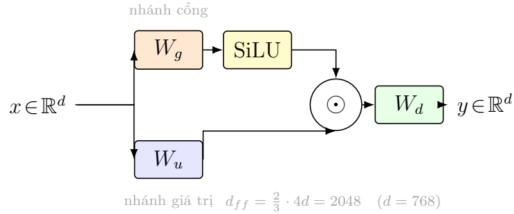
Hình 2.4: Cấu trúc cổng SwiGLU [16].
