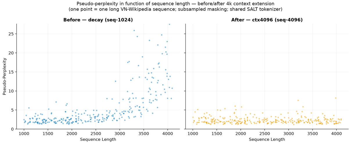
Hình 4.6: Pseudo-perplexity theo độ dài chuỗi trước (trái) và sau (phải) pha mở rộng ngữ cảnh 4.096 token.
