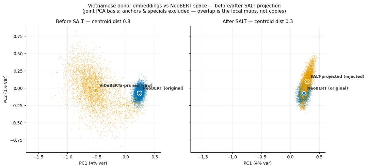
Hình 4.1: Phân bố nhúng của từ vựng tiếng Việt so với không gian NeoBERT trước (trái) và sau (phải) phép chiếu SALT.
