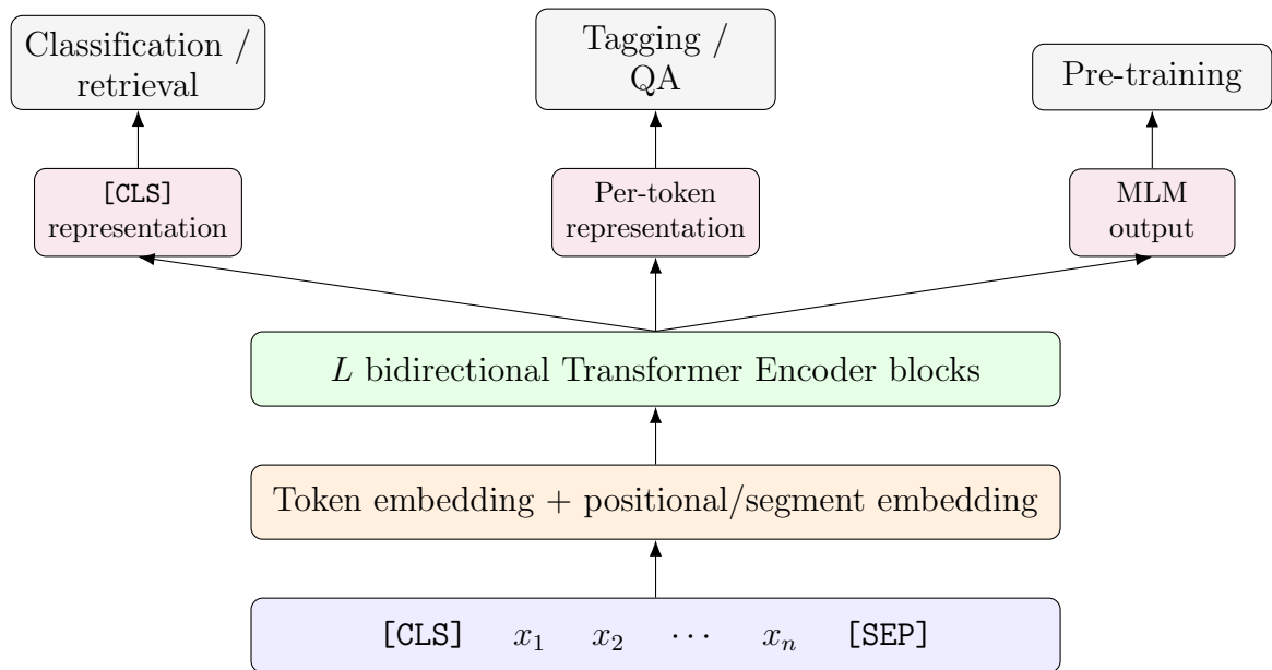
Hình 2.1: Luồng xử lý của một mô hình Encoder-only kiểu BERT.
