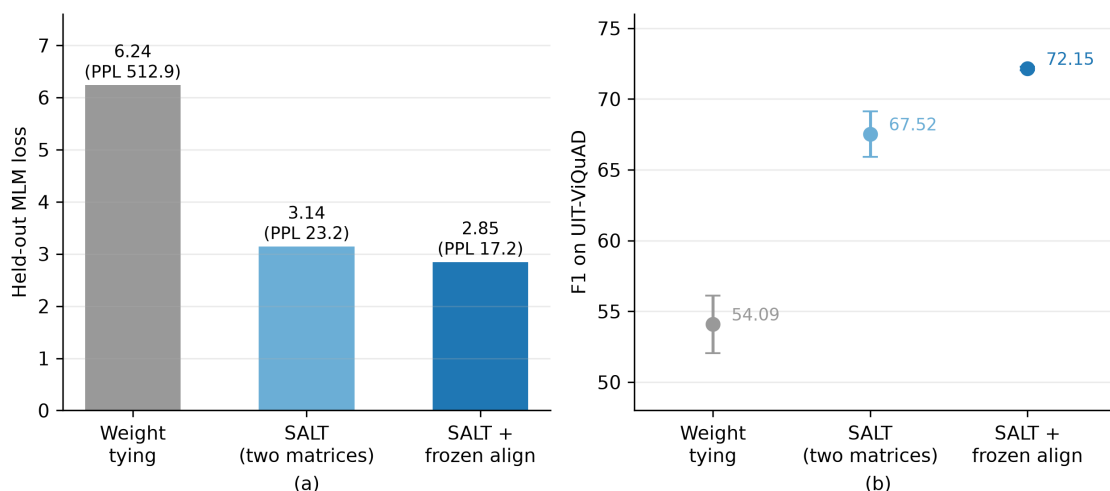
Hình 4.3: So sánh ba chiến lược khởi tạo tại cùng mốc \sim 100 triệu token CPT.
