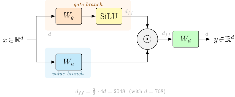
Hình 2.4: Cấu trúc cổng SwiGLU [16]. Nhánh cổng (qua phi tuyến SiLU) điều tiết theo từng phần tử luồng thông tin của nhánh giá trị trước khi chiếu về chiều gốc.
