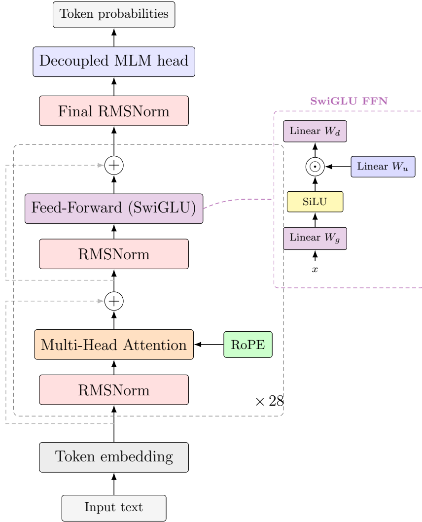
Hình 2.2: Kiến trúc NeoBERT [5].
