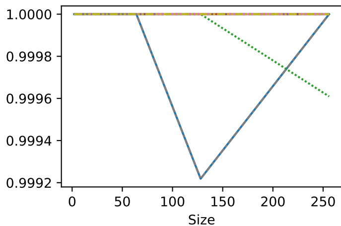
Float-0:0.0001
