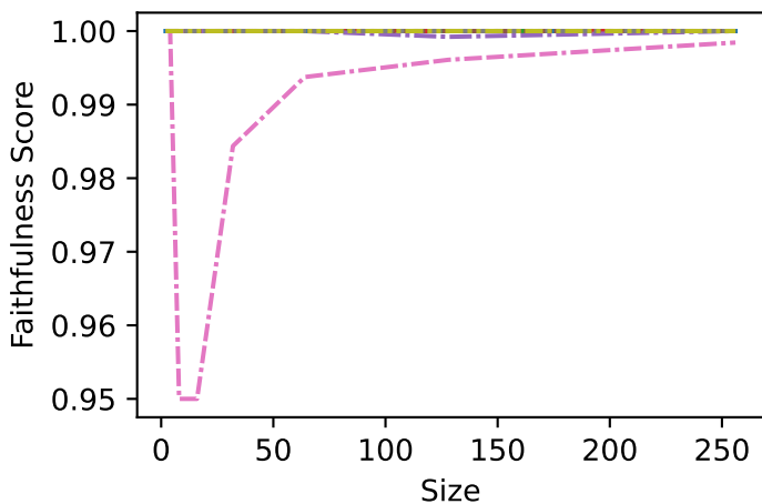
Float-n1000-1000
