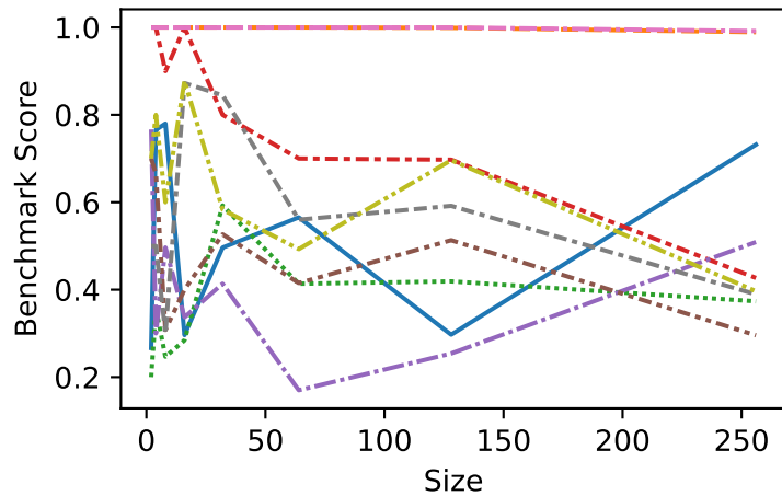
ascii
