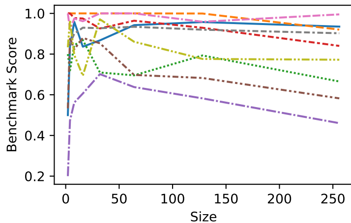
AsCii
