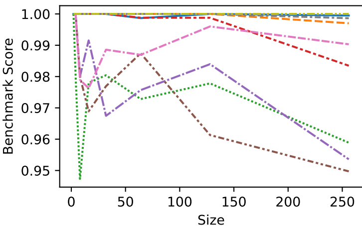
Float-n1000-1000
