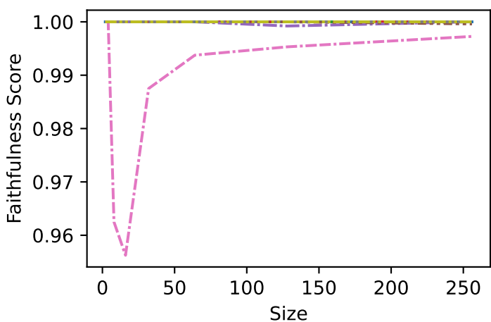
Float-n1000-1000
