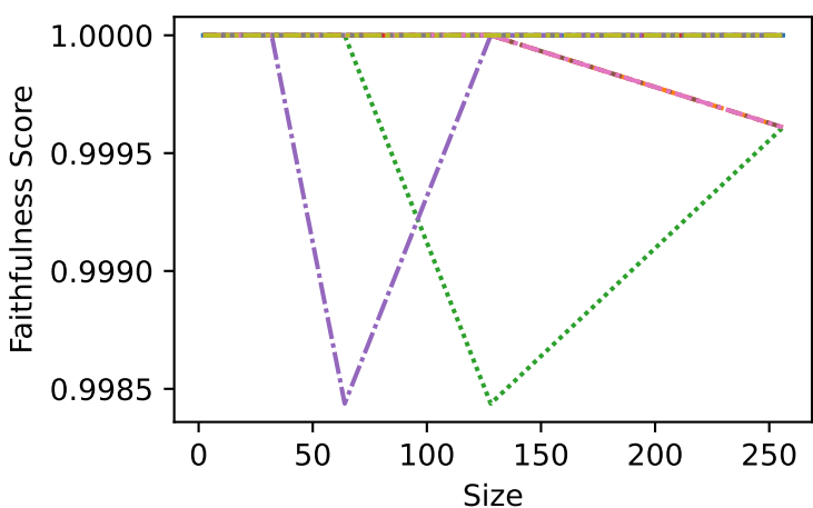
Float-n1000-1000
