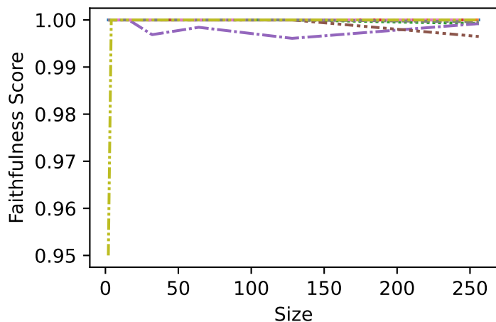
ascii
