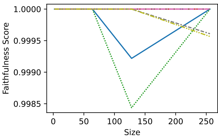
Float-0:0.0001
