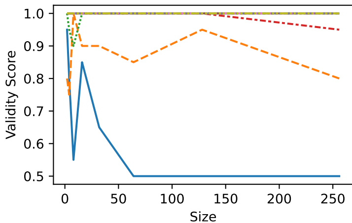
PrfxEnglish
