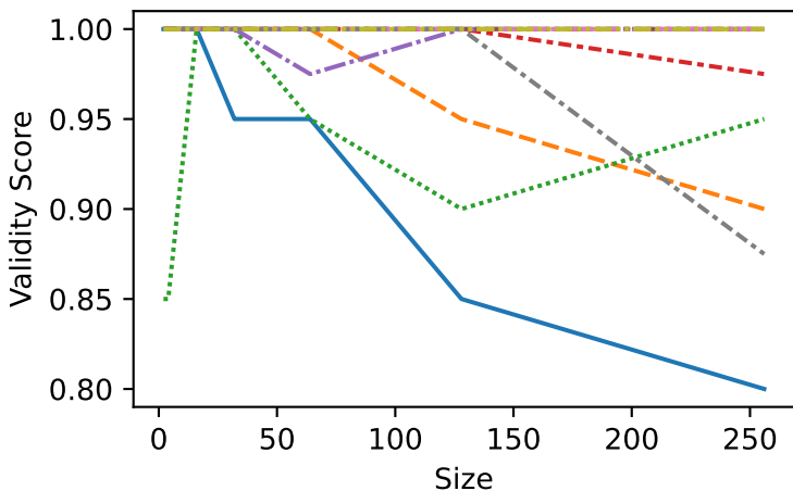
Float-n1000-1000
