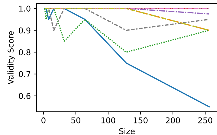
Float-0:0.0001
