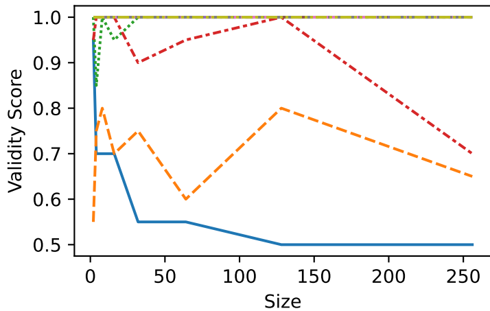
AsCil
