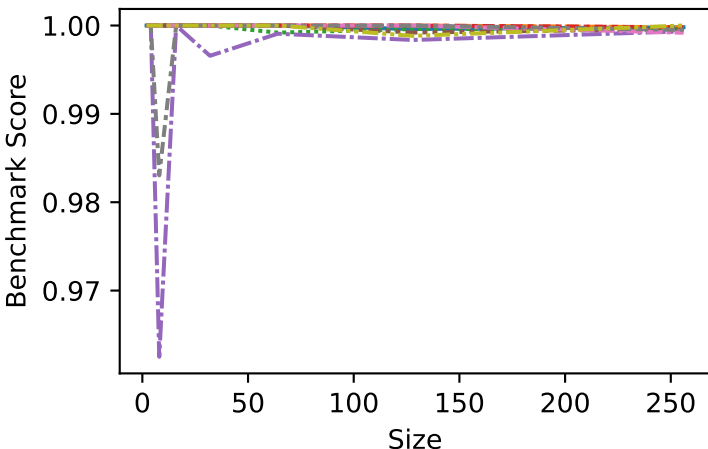
Float-0:0.0001
