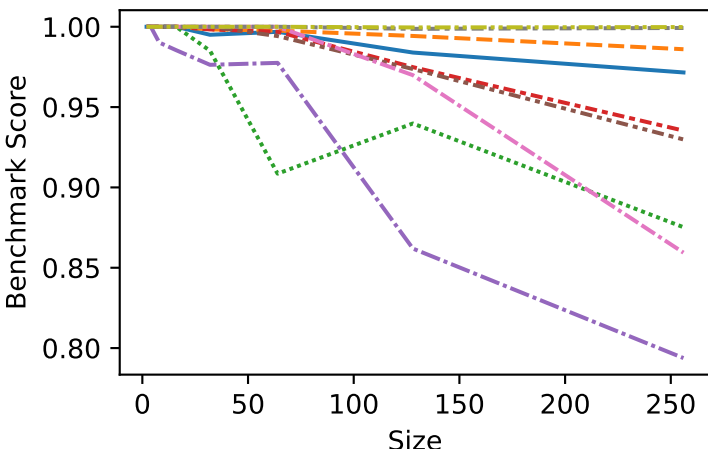
Float-n1000-1000
