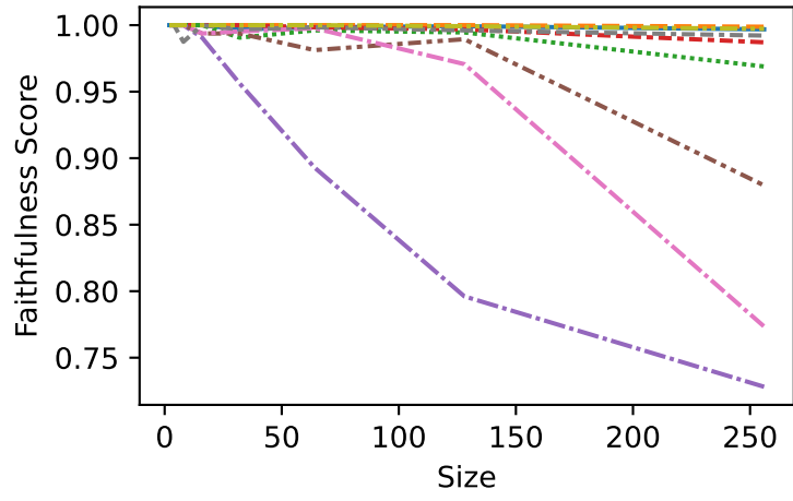
AsCii
