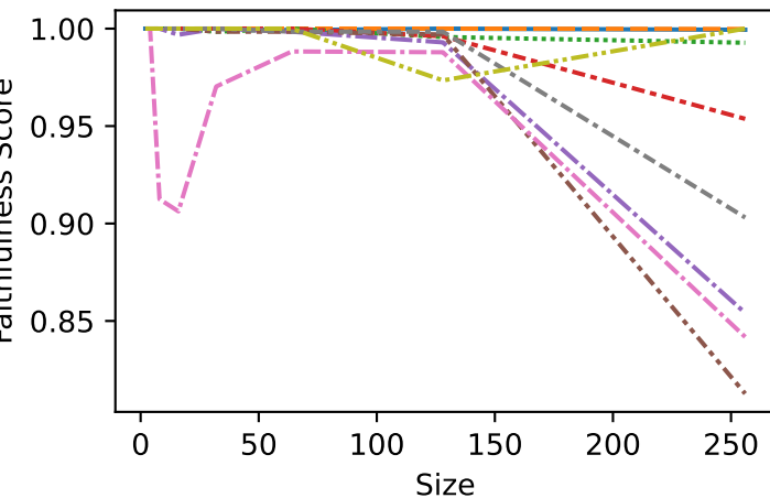
Float-n1000-1000
