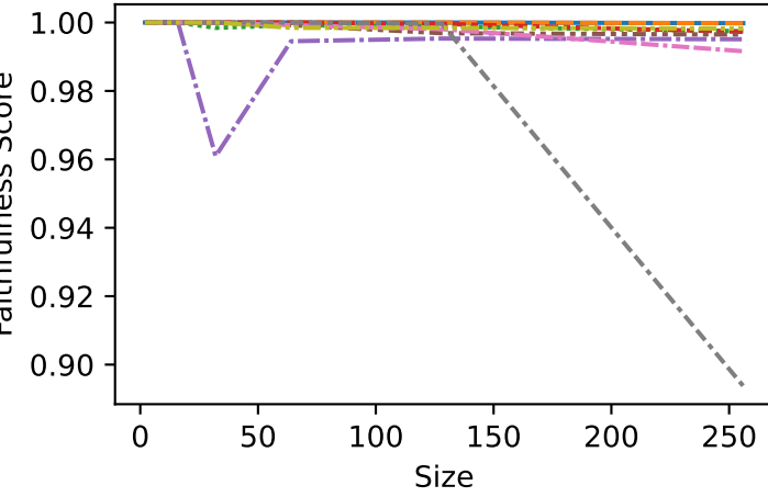
Float-0:0.0001
