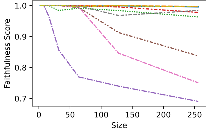
PrfxEnglish
