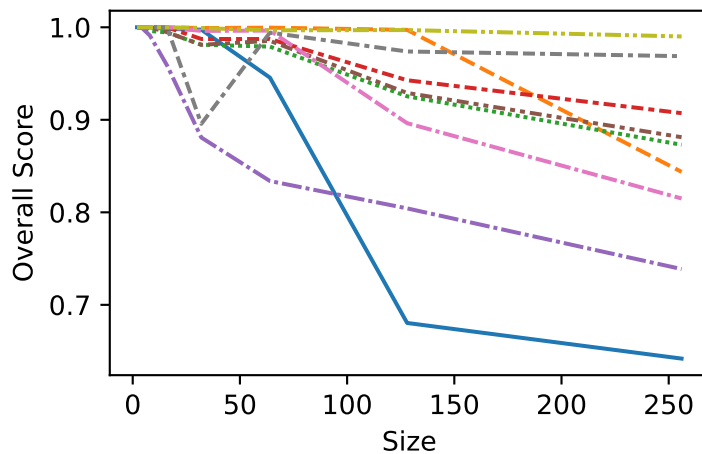
AsCil
