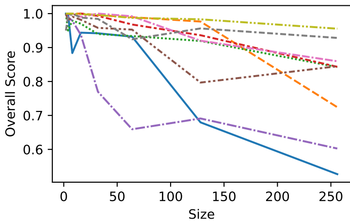
AsCiI
