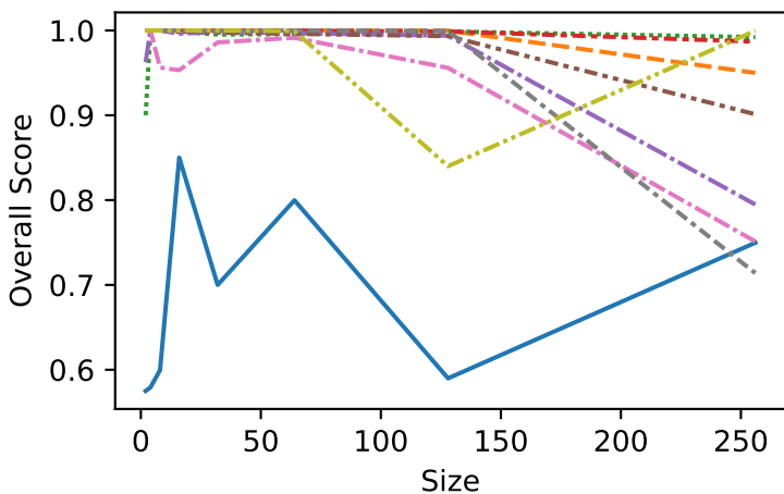
Float-n1000-1000
