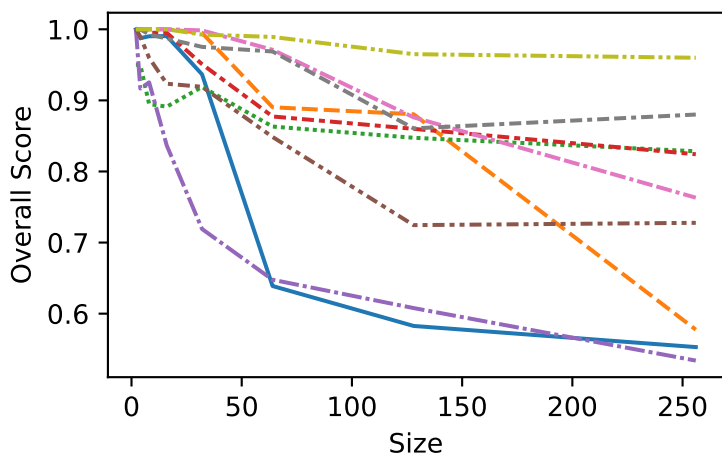
PrfxEnglish
