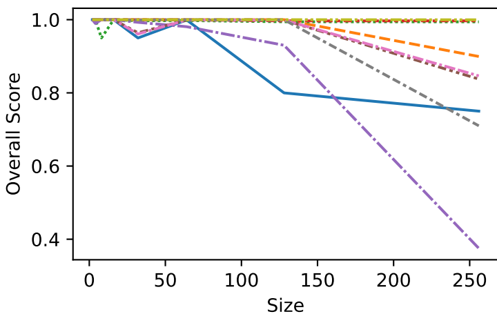
Float-0:0.0001
