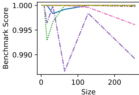
Int-0:1000
