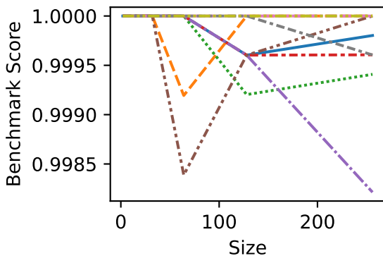
Float-0:1000
