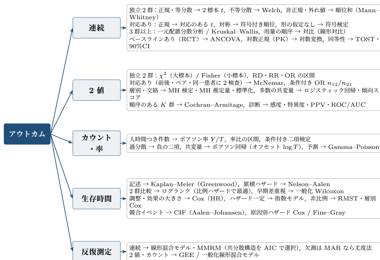
図 A.1 アウトカムからの手法選択
