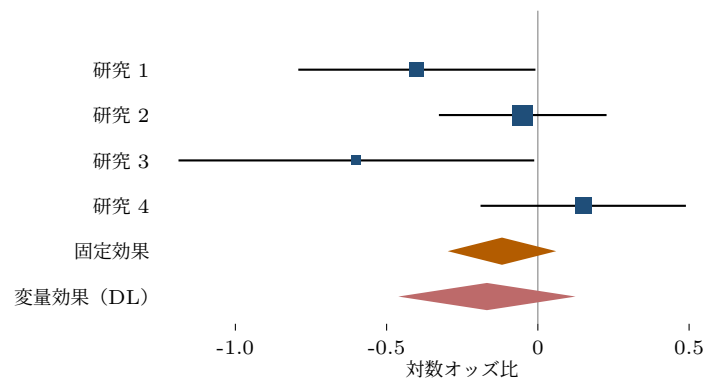
図 15.1 例題 15.1 のフォレストプロット
