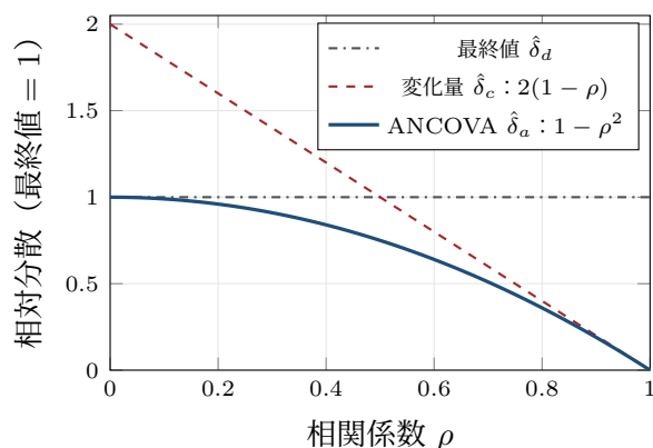
図 8.1 ベースライン調整の 3 推定量の相対分散 (2024 年 医薬 問 2 [5])
