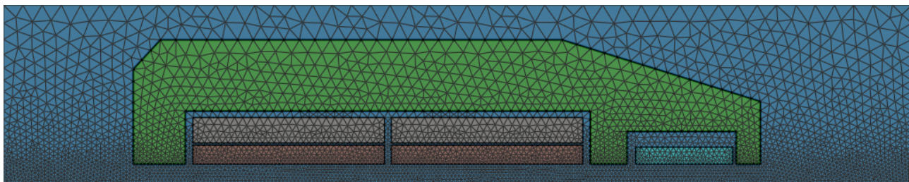
Рисунок Б.2 – Конечноэлементная сетка
