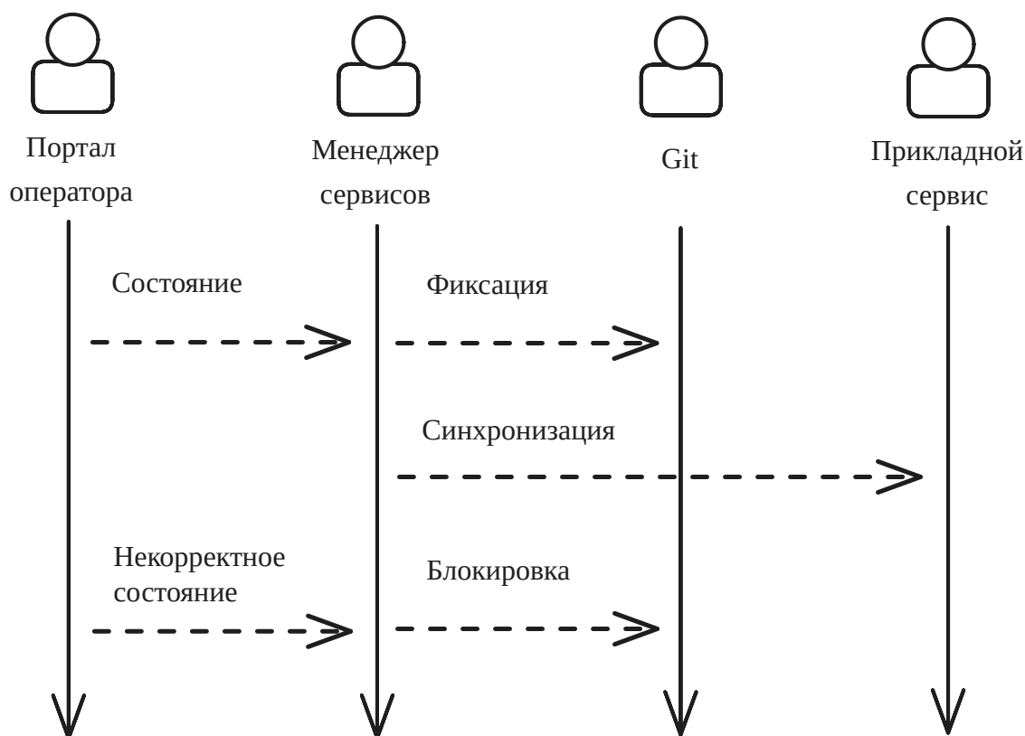
Рисунок 12 – Диаграмма последовательности фиксации состояния
