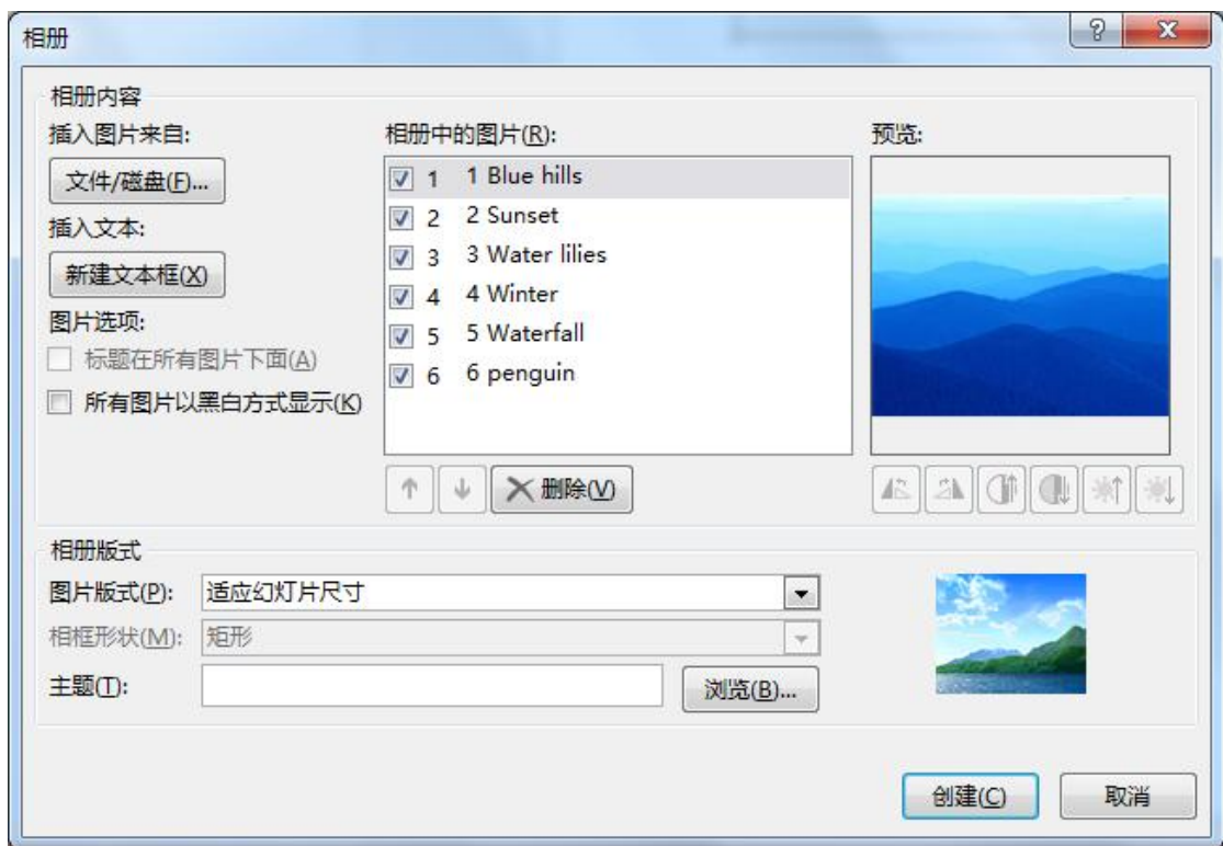
图 3-10 [相册]对话框
