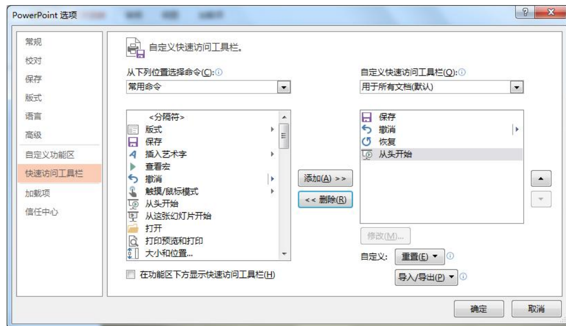
图 3-4 PowerPoint 选项
