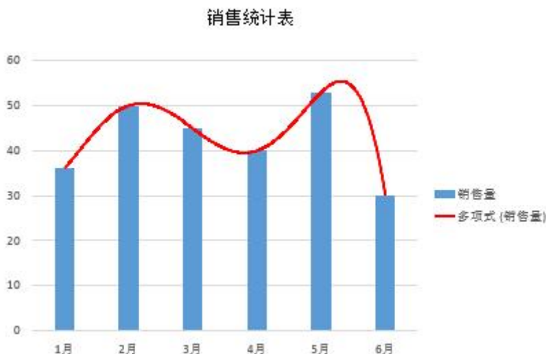
图 3-13 美化趋势线
