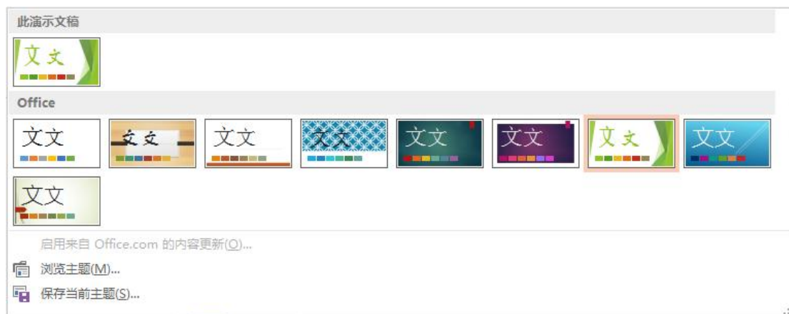
图 3-33 选择主题
