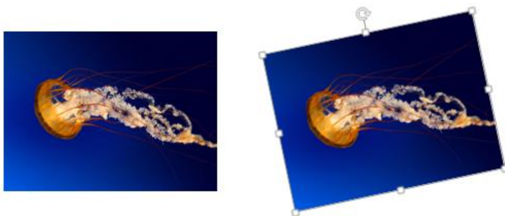
图 3-9 图片的旋转
