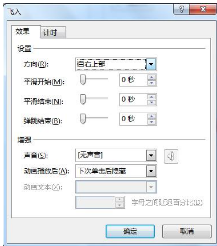
图 3-25 [飞入]对话框
